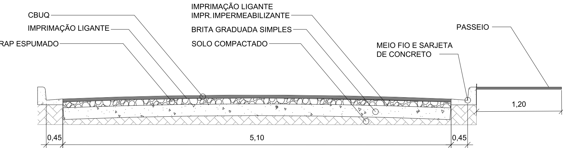
SEÇÃO-TIPO DE PAVIMENTAÇÃO S/ ESC.
