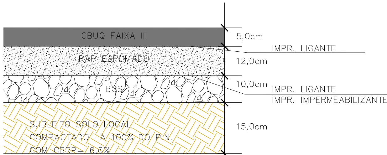
DETALHE - SEÇÃO DE REPARO PROFUNDO S/ ESCALA
