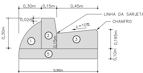
DETALHE DE GUIA E SARJETA 0,45m SEM ESCALA
