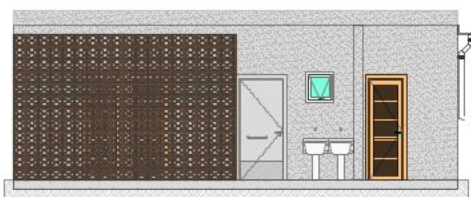
CORTE AA esc. 1:150
