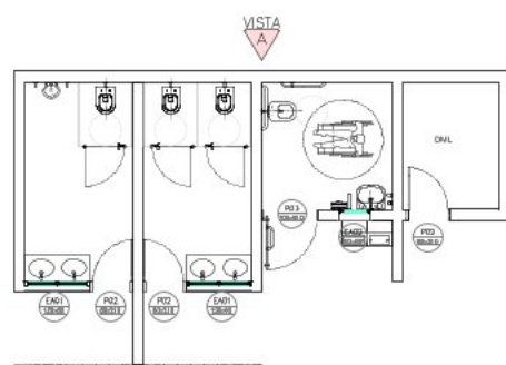
IMPLANTAÇÃO - VEST. 02 esc. 1:150
