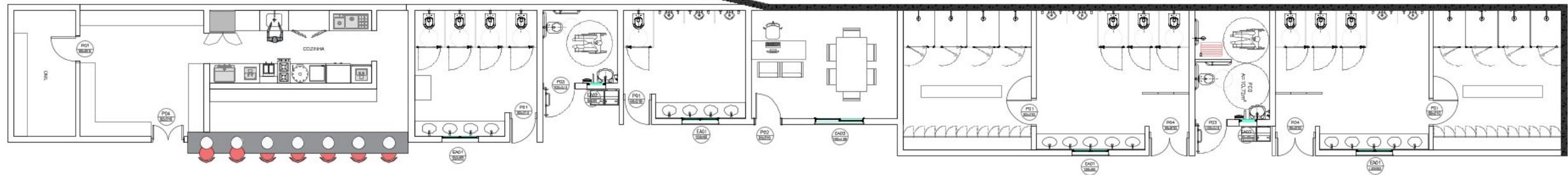
IMPLANTAÇÃO - VEST. 01 esc. 1:150
