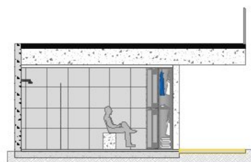
CORTE AA esc. 1:150
