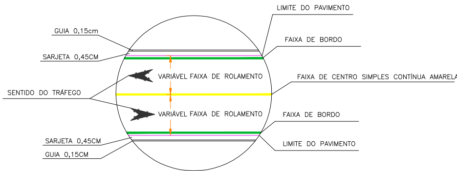
DETALHE DE FAIXA DE ROLAMENTO
