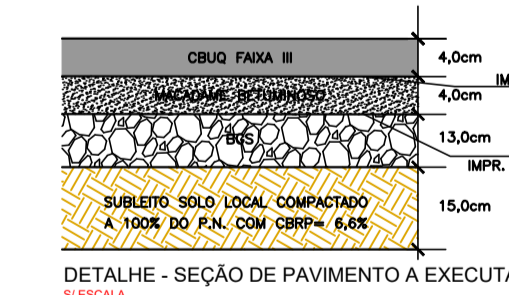
DETALHE - SEÇÃO DE PAVIMENTO A EXECUTAR ESC. 1:25
