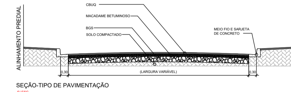
SEÇÃO-TIPO DE PAVIMENTAÇÃO ESC. 1:50
