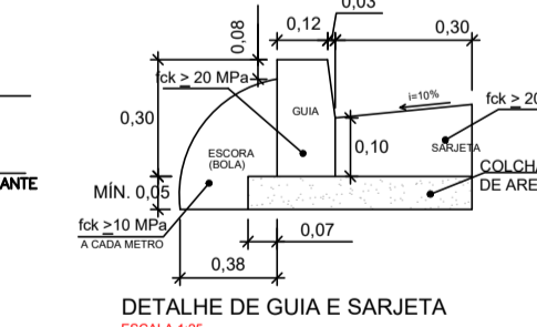
DETALHE DE GUIA E SARJETA ESC. 1:25
