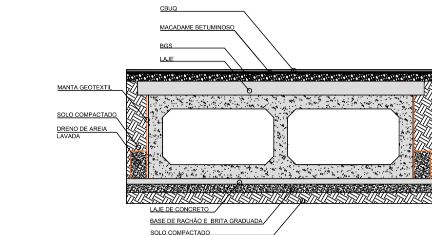
SEÇÃO ADUELA VISTA EM PLANTA ESC. 1:50
