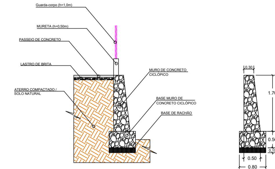
SEÇÃO MURO DE ARRIMO VISTA EM PLANTA ESC. 1:50
