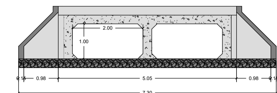
VISTA EM ELEVACÃO ESC. 1:50
