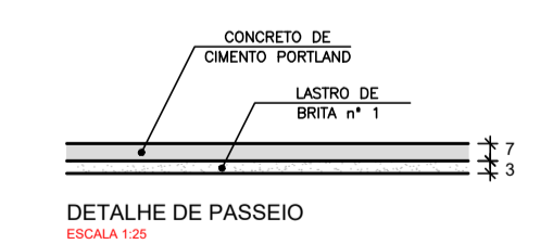
DETALHE DE PASSEIO ESC. 1:25
