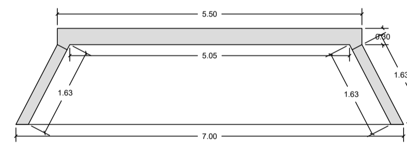
MURO DE ALA VISTA EM PLANTA ESC. 1:50
