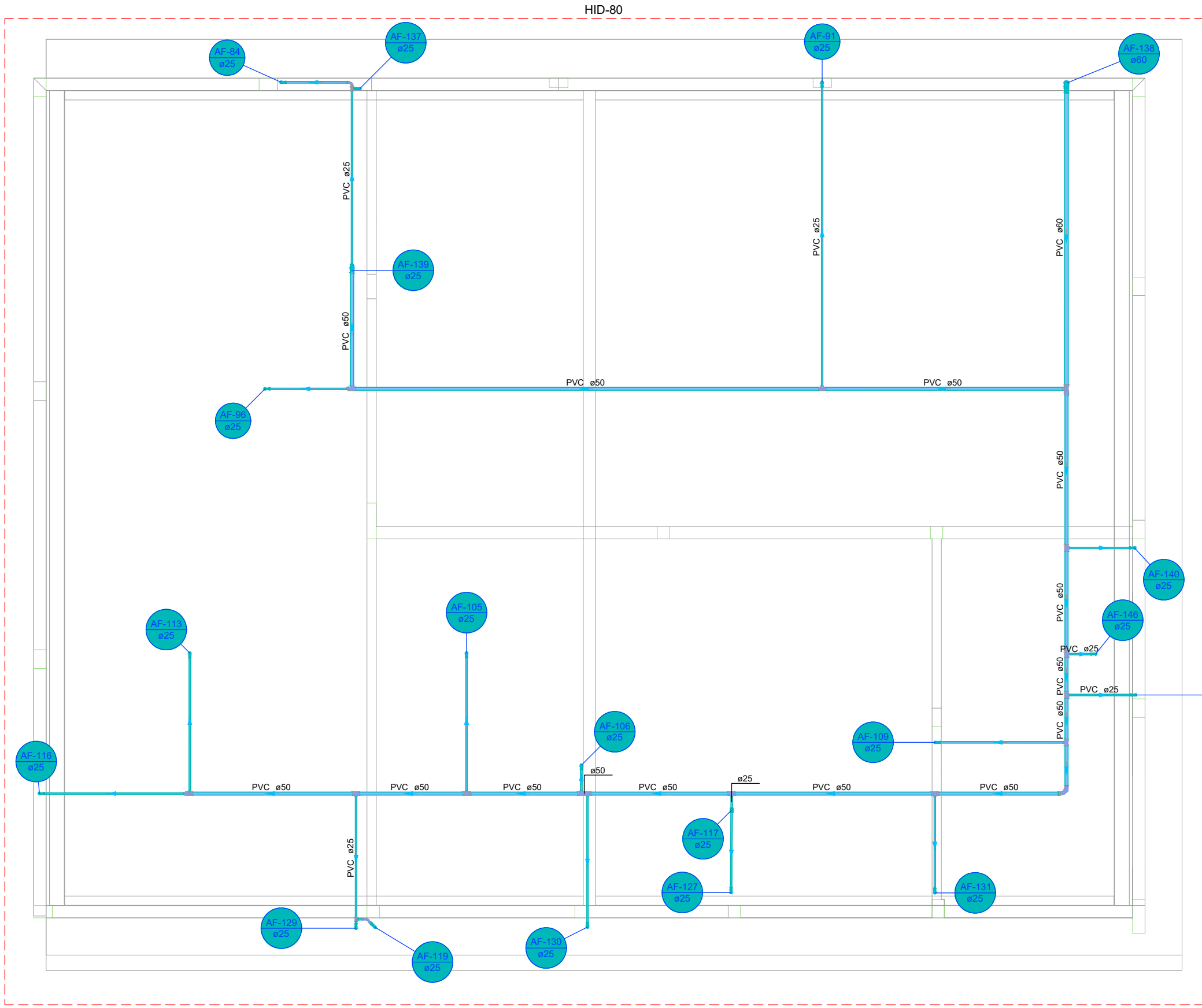
PLANTA - HIDRÁULICO - COBERTURA ESC. 1/100
