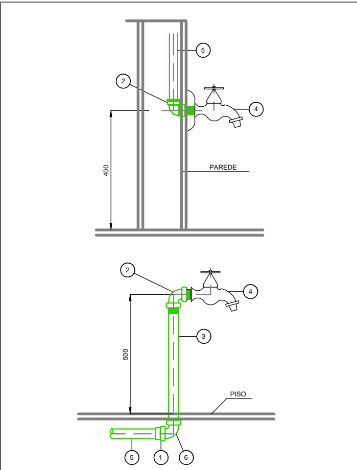
DETALHE TÍPICO DE FIXAÇÃO DE TUBULAÇÃO
