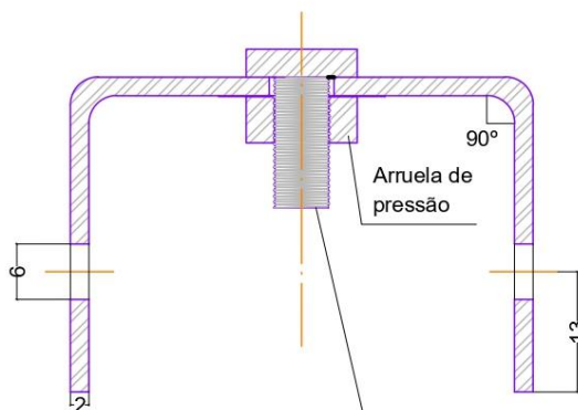
CORTE A-A
