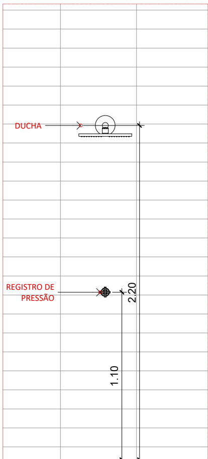
ELEV. TIPO - DUCHA ARENA CAMPANÁRIO ESC. 1:25
