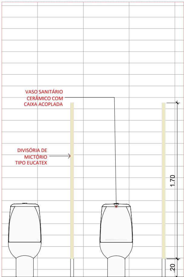
ELEV. TIPO - SANITÁRIOS ARENA CAMPANÁRIO ESC. 1:25
