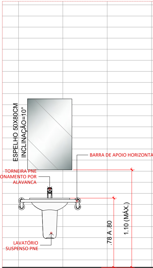
ELEV. TIPO - LAVATÓRIO PNE ARENA CAMPANÁRIO ESC. 1:25
