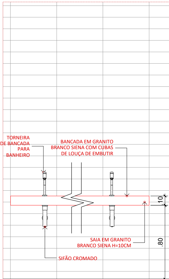
ELEV. TIPO - BANCADA ARENA CAMPANÁRIO ESC. 1:25
