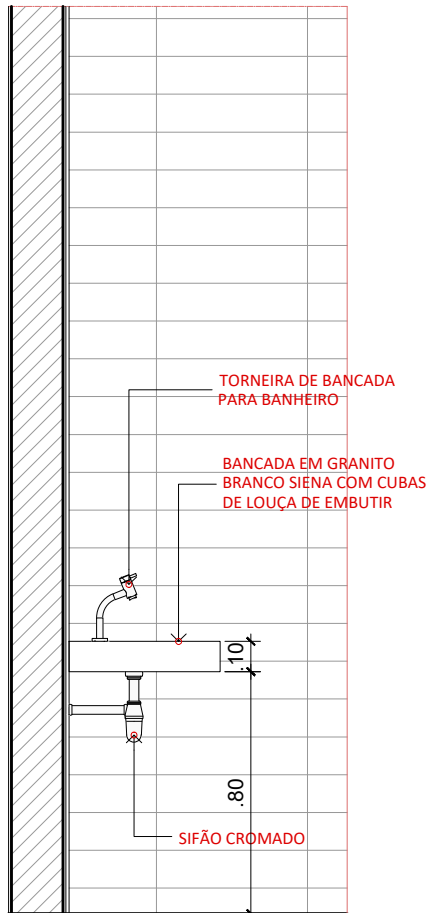
ELEV. TIPO - BANCADA ARENA CAMPANÁRIO ESC. 1:25
