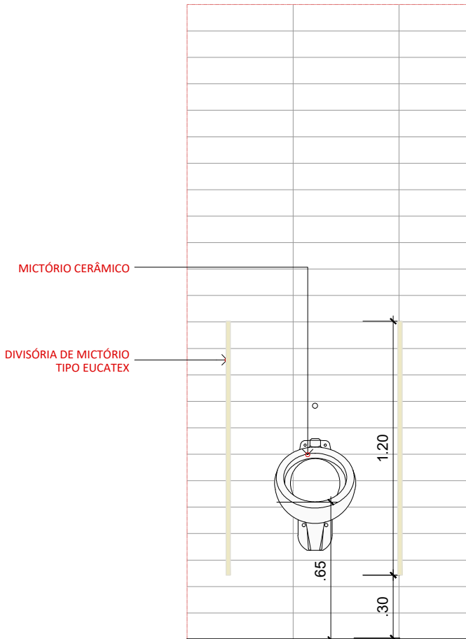
ELEV. TIPO - MICTÓRIOS ARENA CAMPANÁRIO ESC. 1:25
