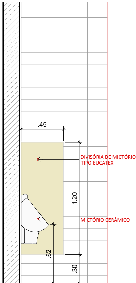
ELEV. TIPO - MICTÓRIOS ARENA CAMPANÁRIO ESC. 1:25
