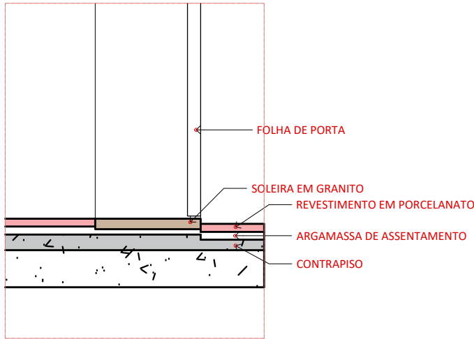
DETALHE TIPO - SOLEIRA ARENA CAMPANÁRIO ESC. 1:10
