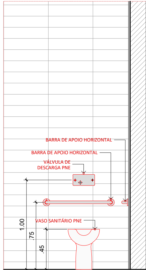
ELEV. TIPO - VASO PNE ARENA CAMPANÁRIO ESC. 1:25
