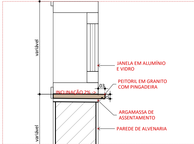
DETALHE TIPO - PEITORIL ARENA CAMPANÁRIO ESC. 1:10
