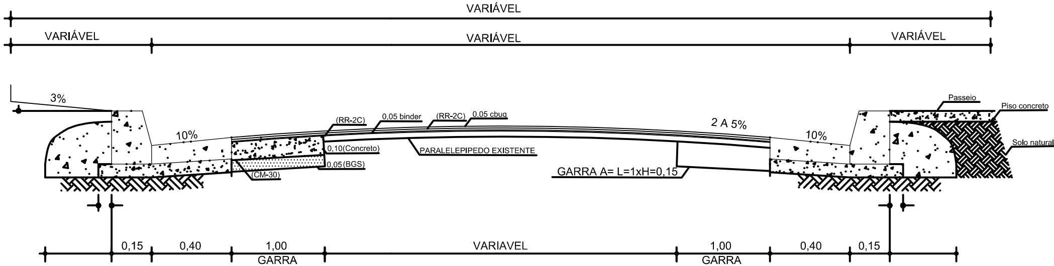
SEÇÃO TIPO I SEÇÃO TIPO RECAPEAMENTO SEM ESCALA
