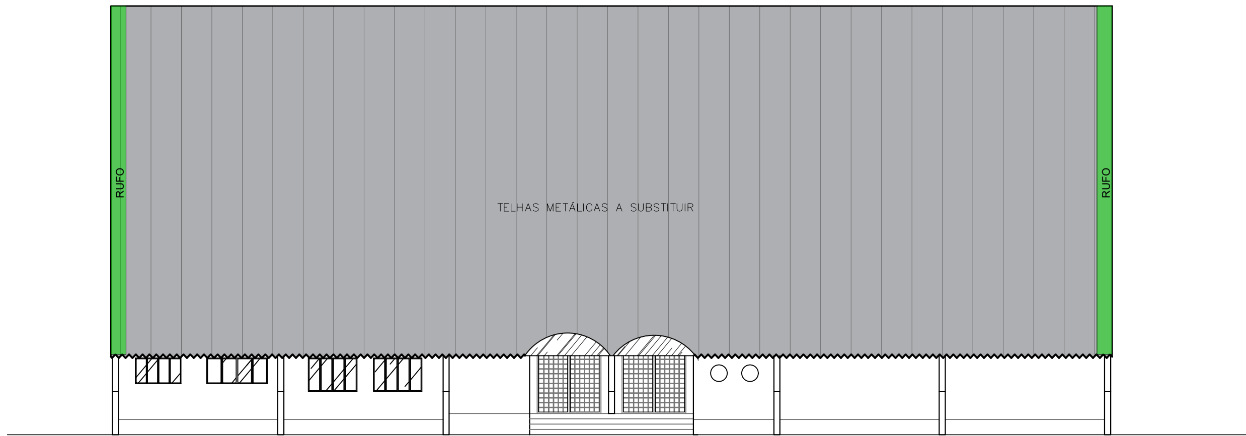
4 FACHADA 1 PLANTA ARQUITETÔNICA ESCALA 1:125
