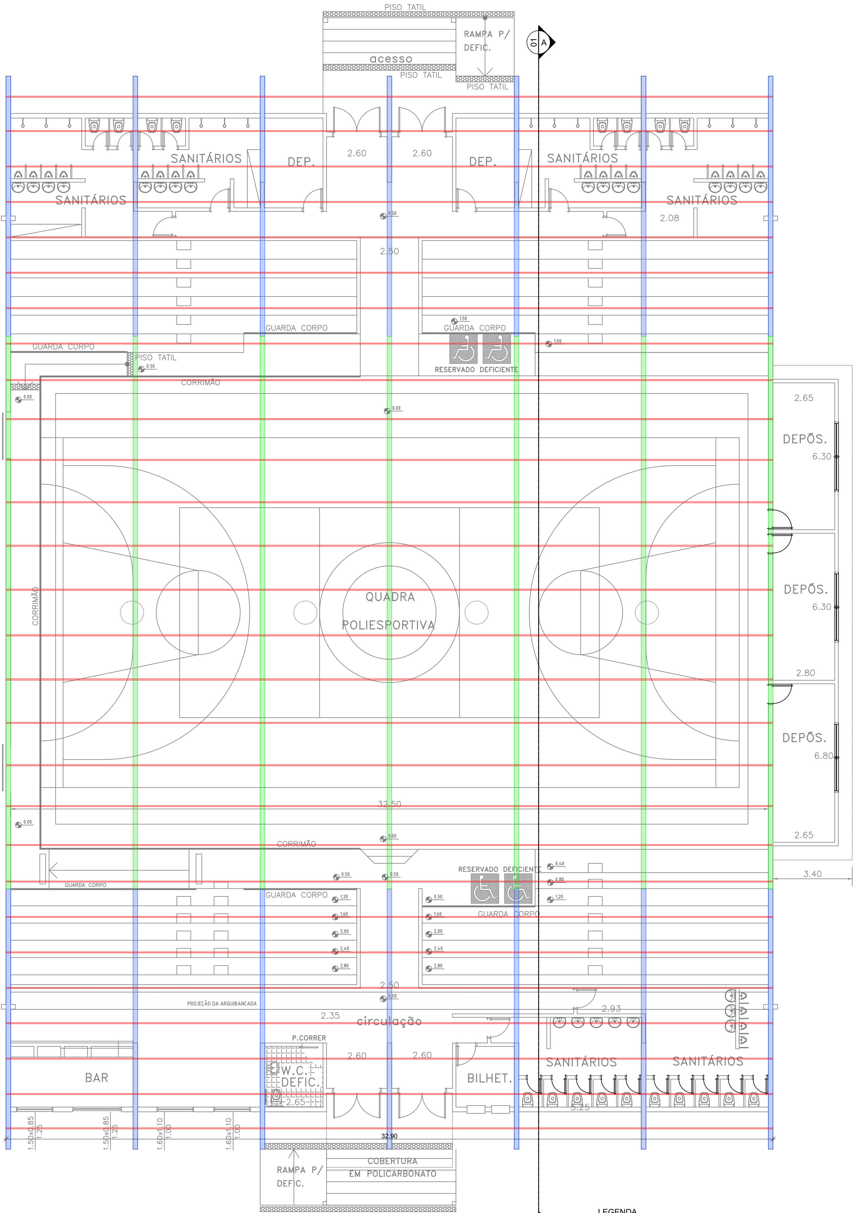
1 PLANTA DA ESTRUTURA DA COBERTURA PLANTA ARQUITETÔNICA ESCALA 1:100
