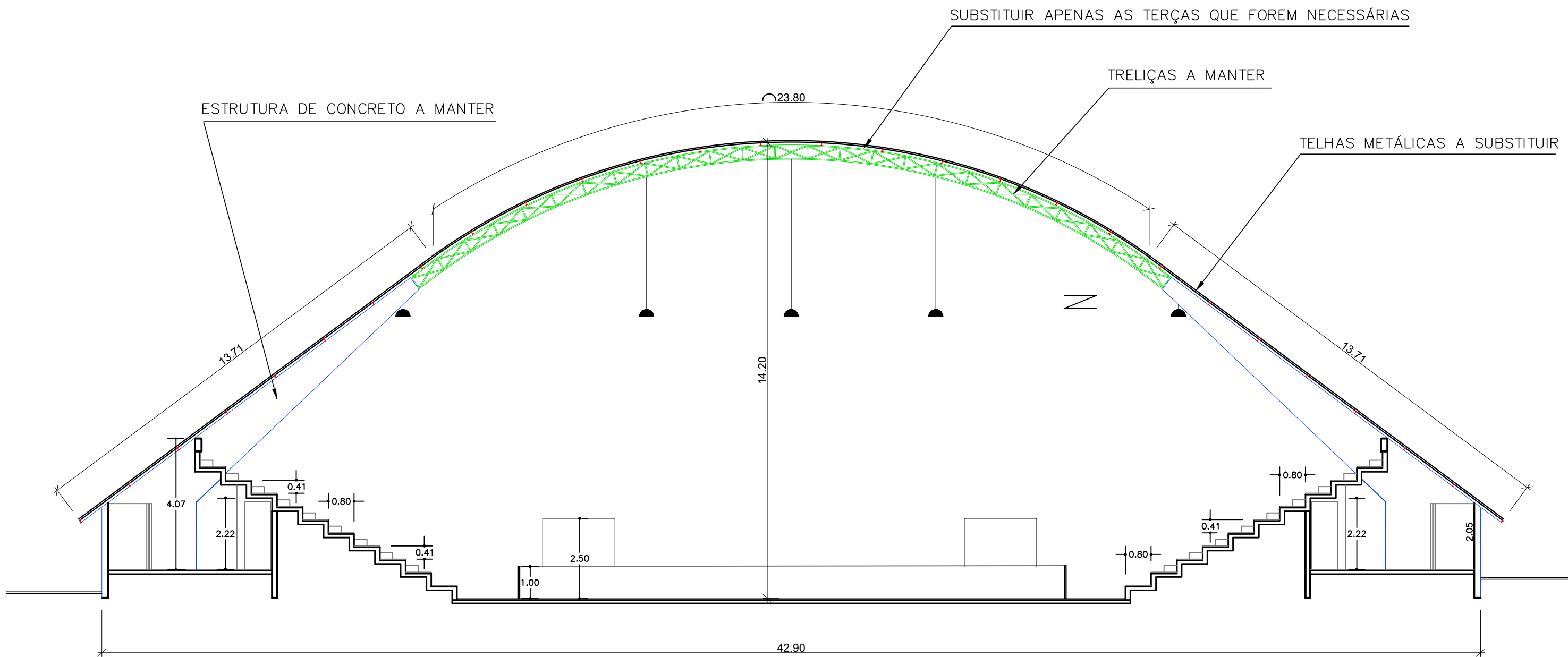
3 CORTE A-A PLANTA ARQUITETÔNICA ESCALA 1:125
