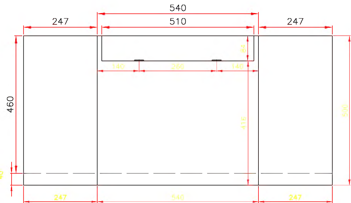
ELEVAÇÃO CABECEIRA (02x) ESCALA 1:75
