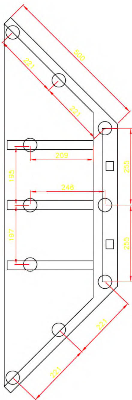
LOCAÇÃO DAS ESTACAS (2x) ESCALA 1:75
