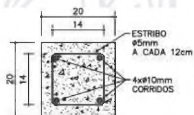
VIGA BALDRAME
