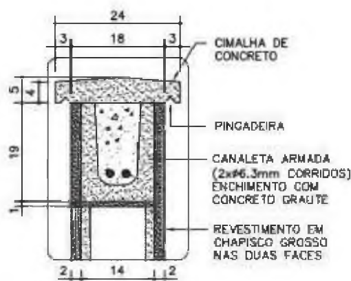
DET. 01
