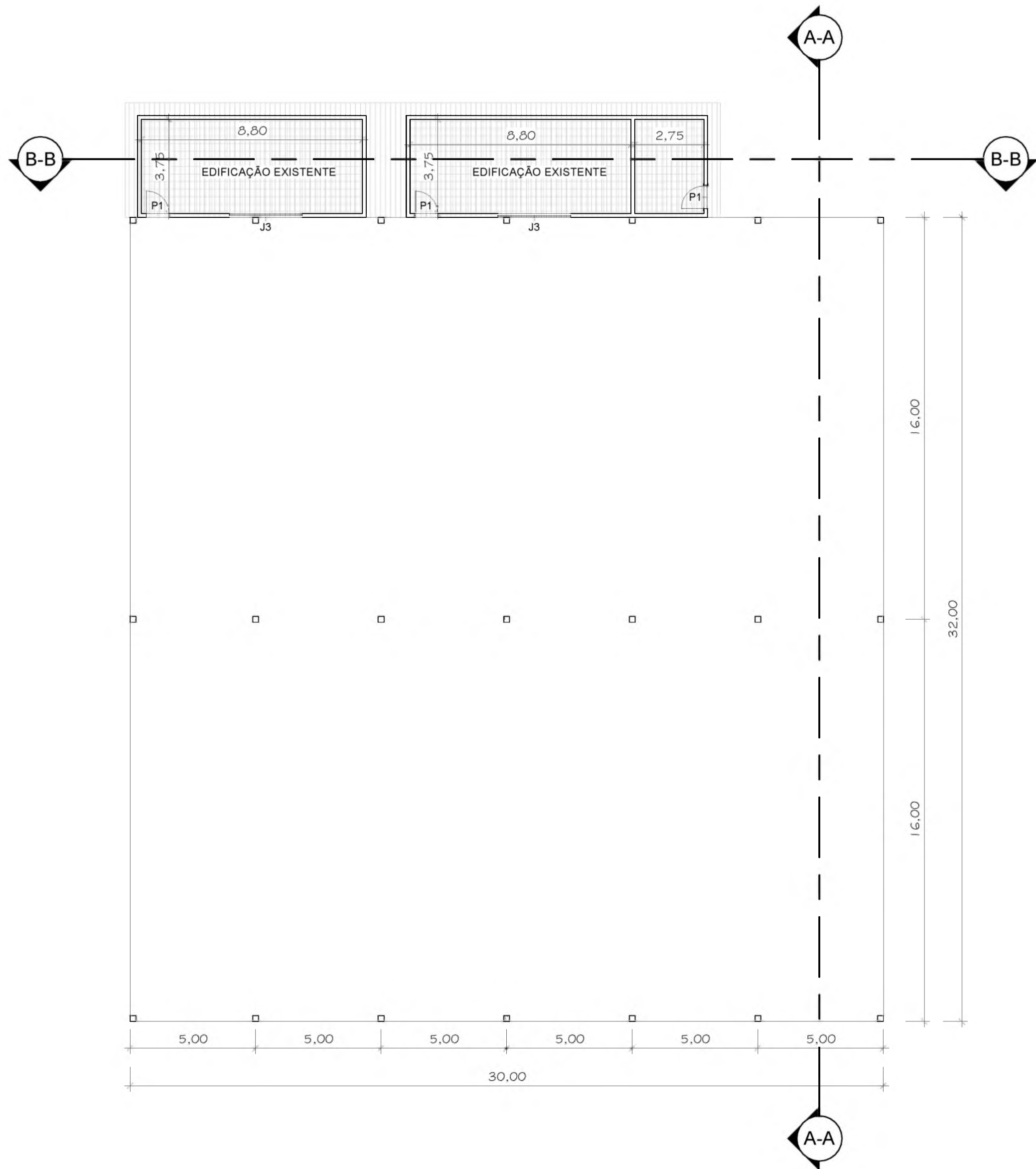
1 TÉRREO 1 : 150
