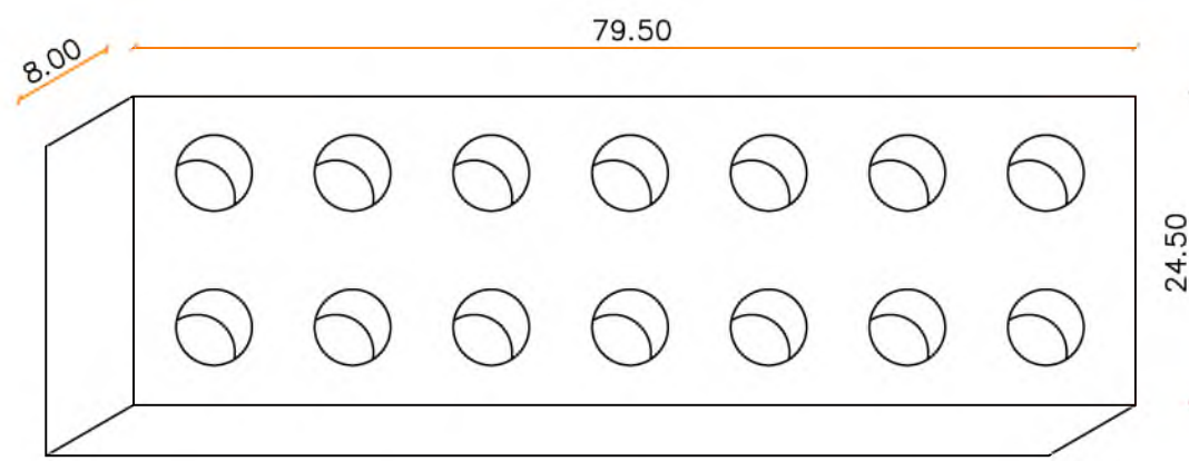
Detalhe "A" - Grelha em Concreto Pré moldada Medidas em centímetros
