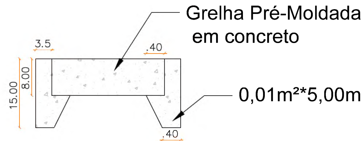
Detalhe "B" - Canaleta em duas peças para apoio de grelha. Medidas em centímetros
