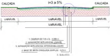
SEÇÃO TRANSVERSAL PAVIMENTAÇÃO ASFÁLTICA
