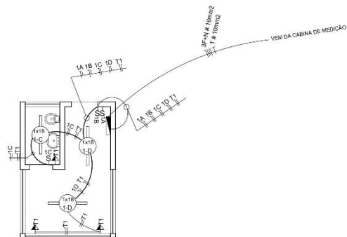
PORTARIA - ELÉTRICA ESCALA 1:50
