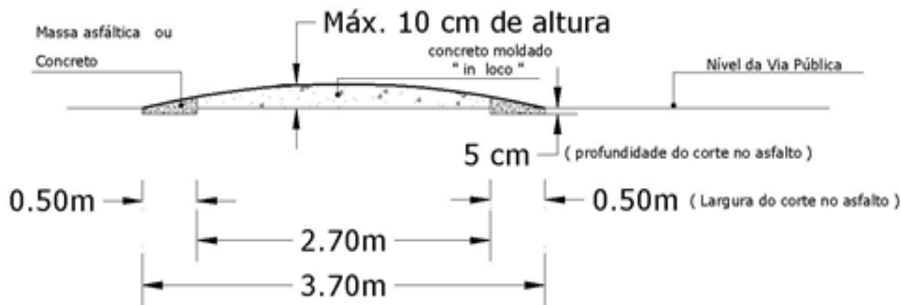
Lombada - Corte Transversal Esquemático
