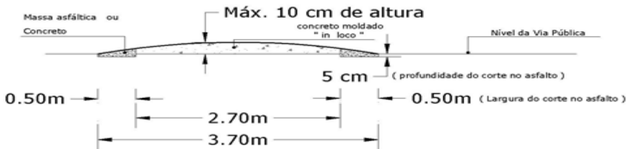
Lombada - Corte Transversal Esquemático
