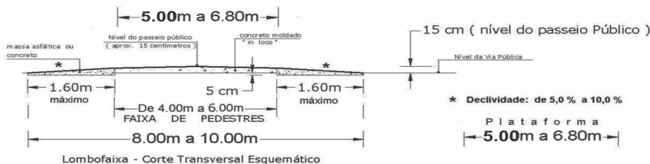
Lombofaixa - Corte Transversal Esquemático
