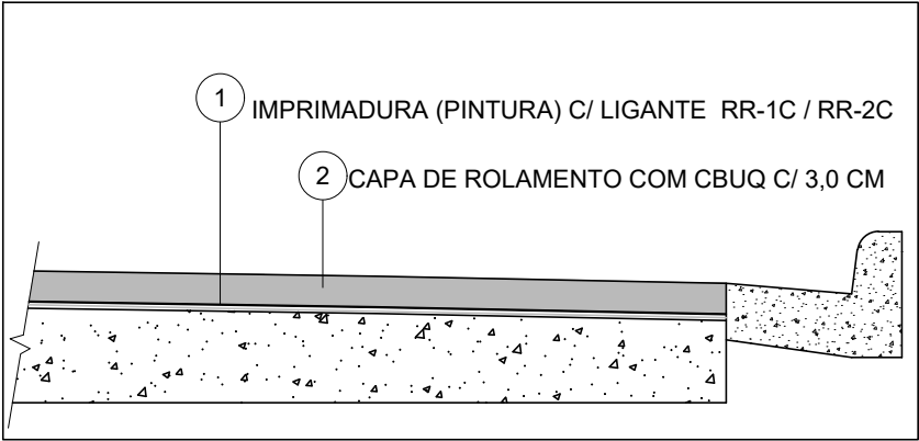
CORTE TRANSVERSAL DA CAPA ASFÁLTICA
