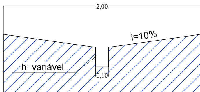
Corte A-A
