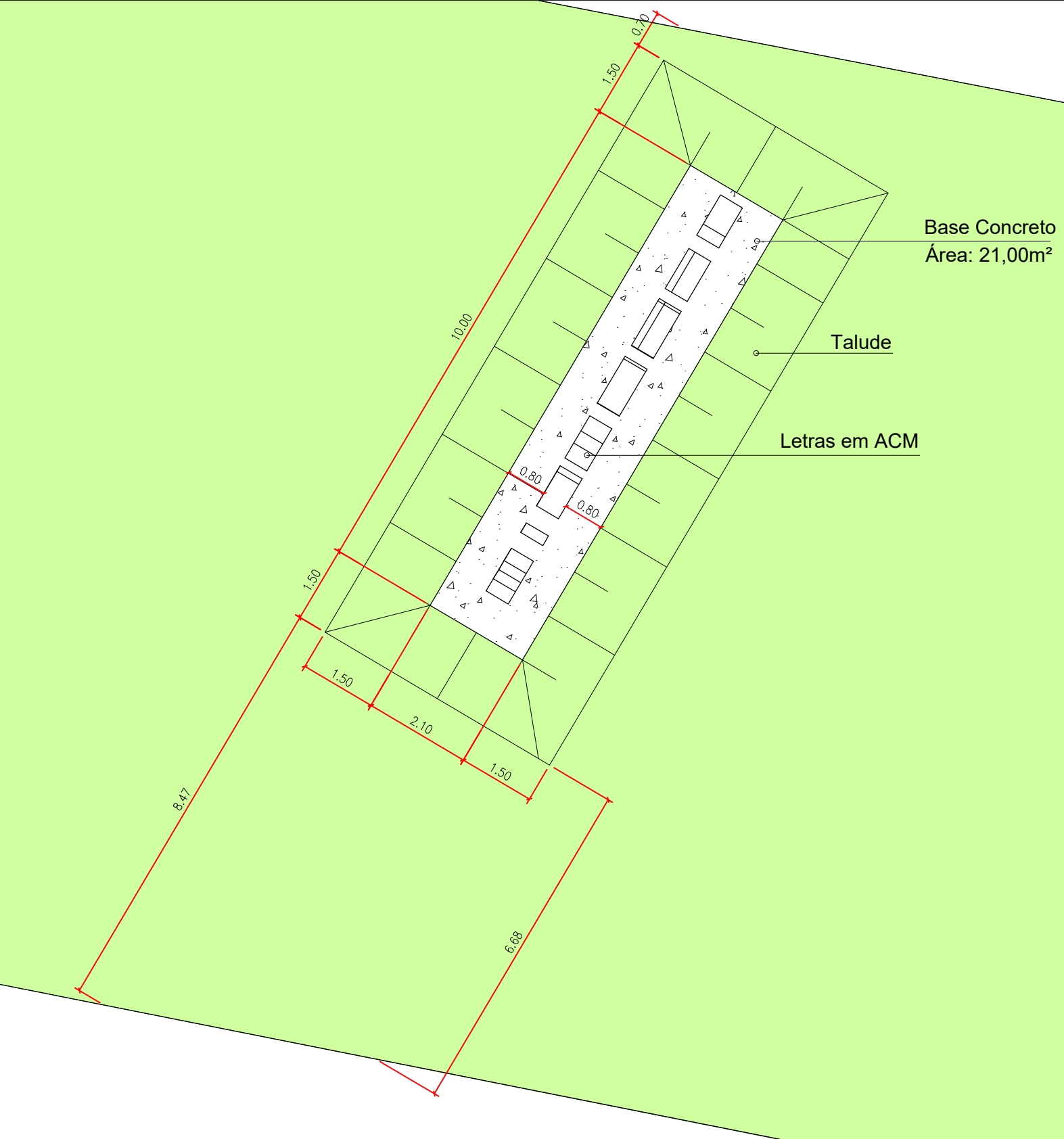
PROJETO PLANTA BAIXA LETREIRO ESC. 1:100
