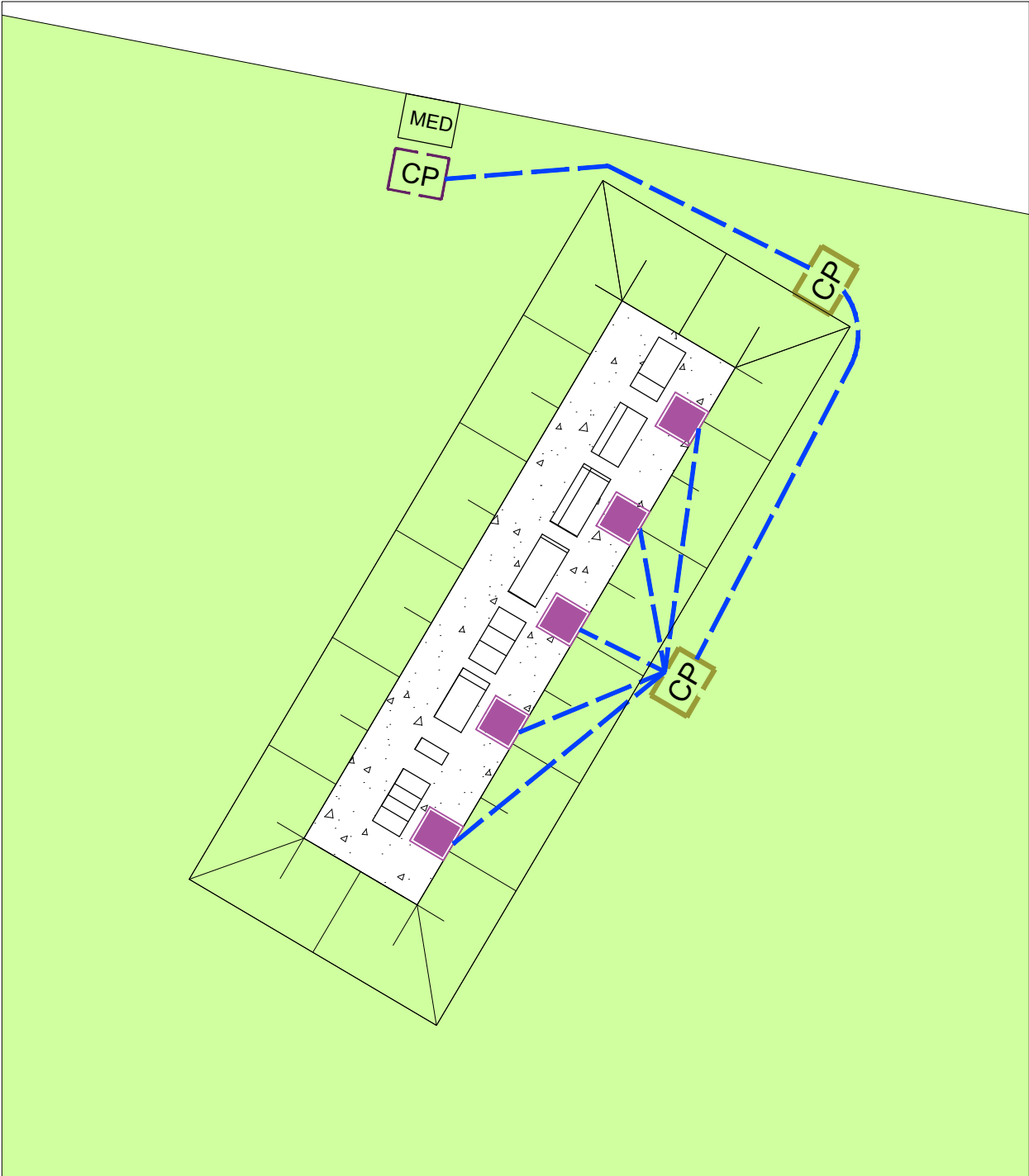
PROJETO ILUMINAÇÃO LETREIRO ESC. 1:100
