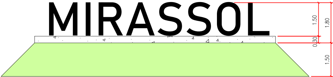
PROJETO VISTA ILUMINAÇÃO LETREIRO ESC. 1:100
