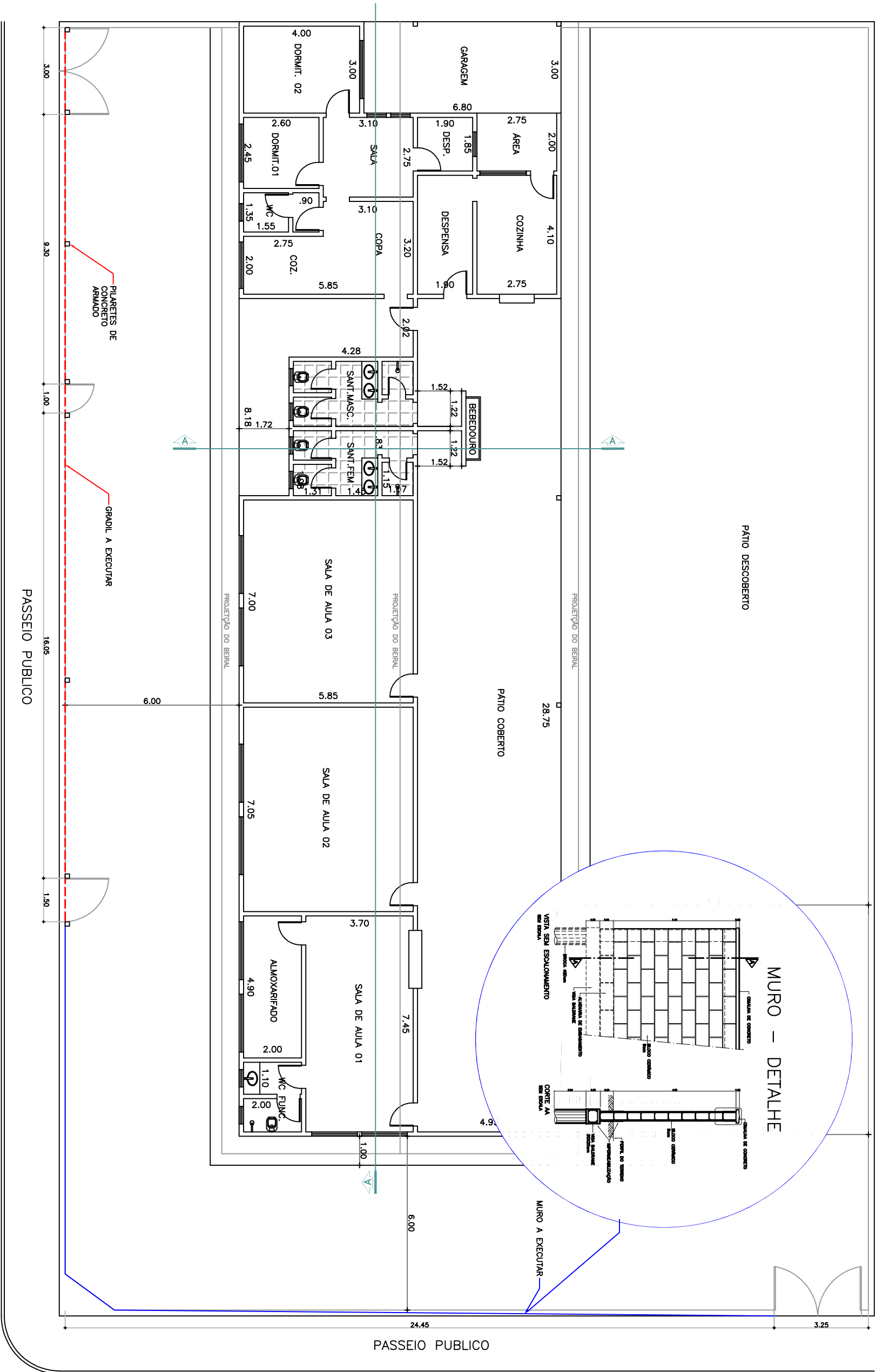
PLANTA BAIXA ESC: 1:100
