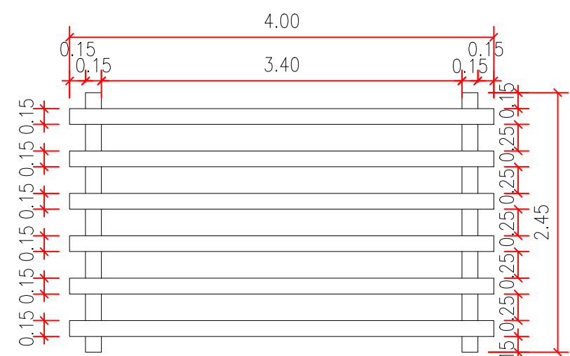
PLANTA BAIXA
