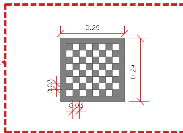
DETALHAMENTO TABULEIRO MESA ESC. 1:10
