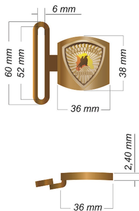
FIVELA PARTE MACHO
