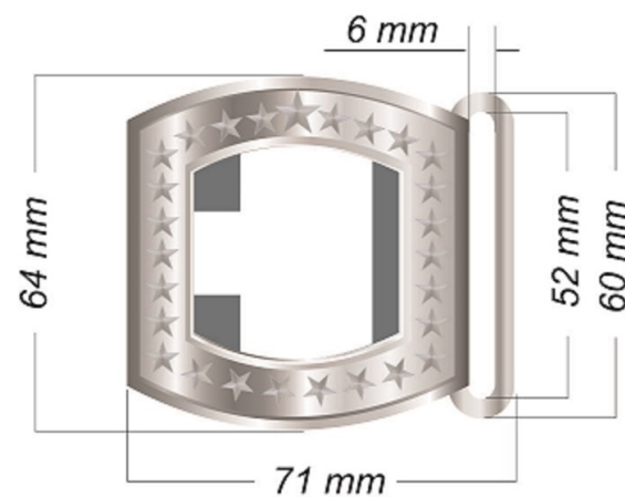
FIVELA PARTE FÊMEA
