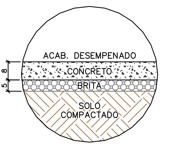
DETALHE GÊNÉRICO PASSEIO EM CONCRETO NÃO ARMADO Medidas em centímetros ESCALA 1:10
