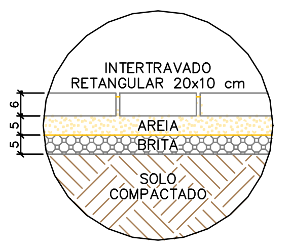
DETALHE GÊNÉRICO PISO INTERTRAVADO Medidas em centímetros ESCALA 1:10
