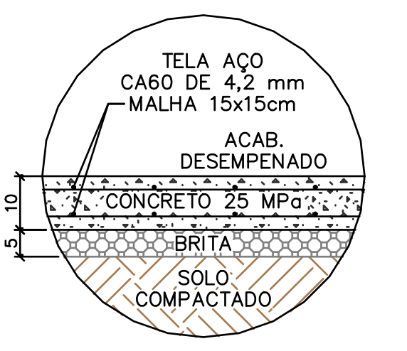
DETALHE GÊNÉRICO BASE DE CONCRETO ARMADO COM TELA Q-92 Medidas em centímetros ESCALA 1:10
