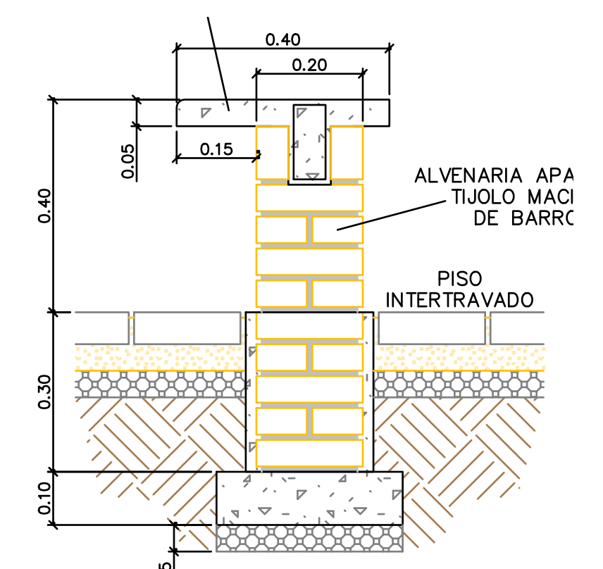
BANCO EM ALVENARIA APARENTE MEDIDAS – VER DETALHE EM CADERNO TÉCNICO SIURB ESCALA 1:10
