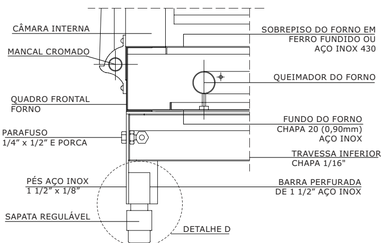
DETALHE C
