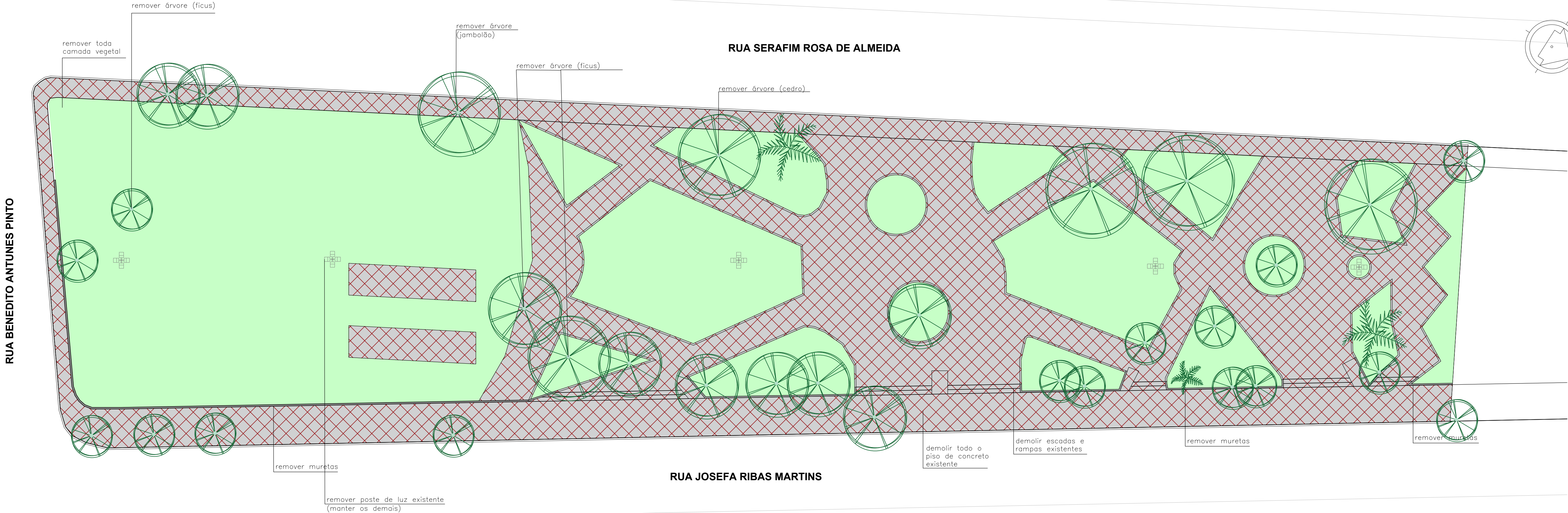
PLANTA DE DEMOLIÇÃO ESCALA 1:200
