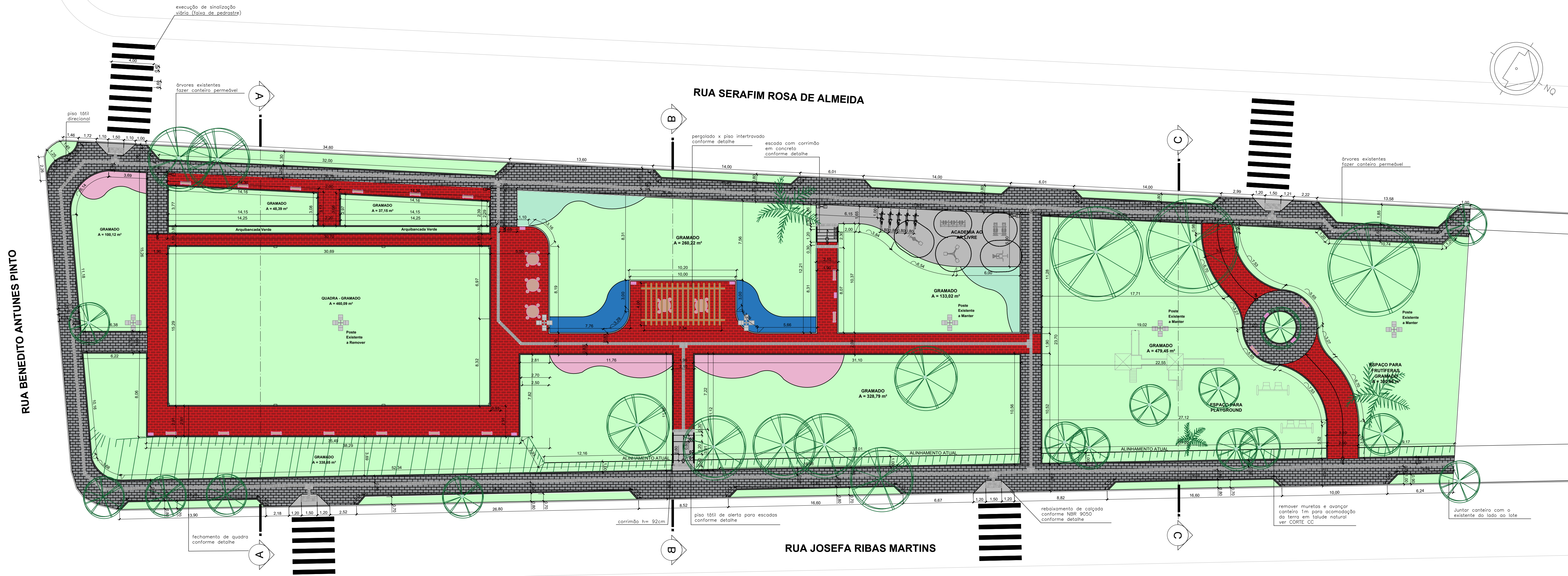
PLANTA DE COTAS - NOVA IMPLANTAÇÃO ESCALA 1:200
