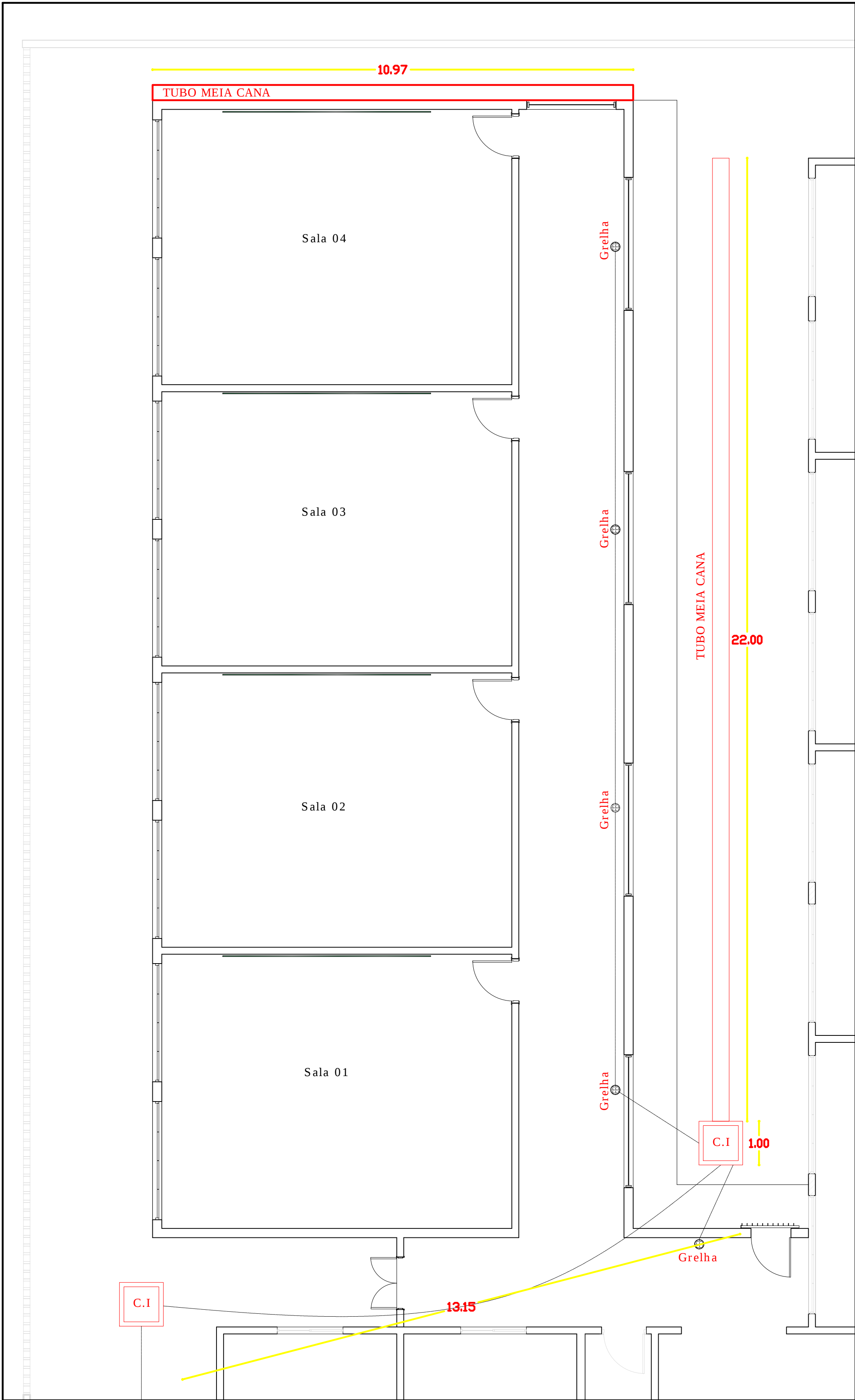
PLANTA DRENAGEM/ESGOTO Esc. 1:100
