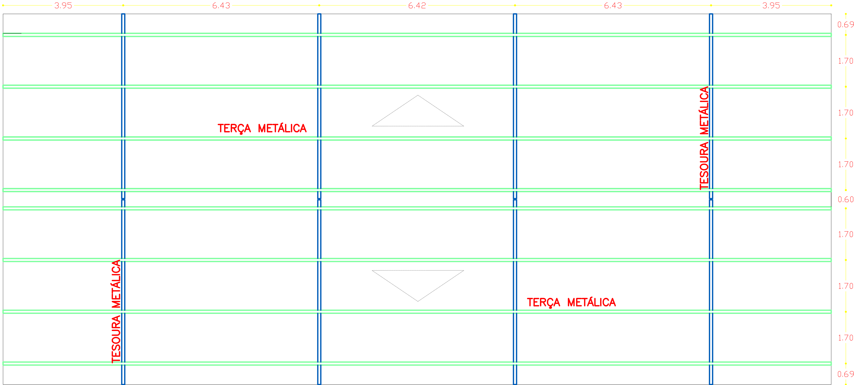
ESTRUTURA COBERTURA SALAS Esc. 1:100
