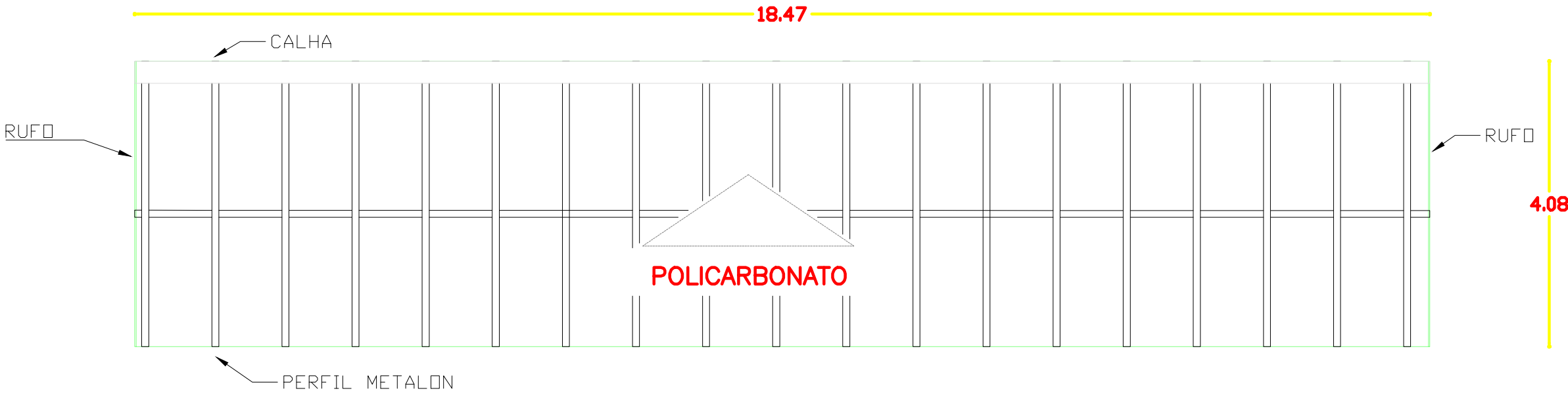
ESTRUTURA COBERTURA HALL Esc. 1:50
