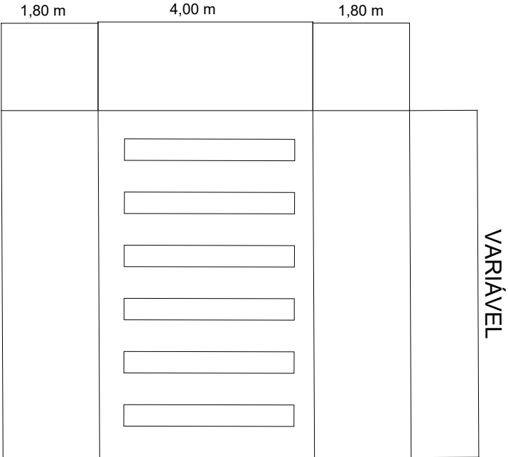
FAIXA ELEVADA SEM ESCALA
