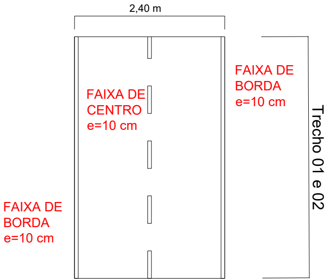
SINALIZAÇÃO DA CICLOVIA SEM ESCALA
