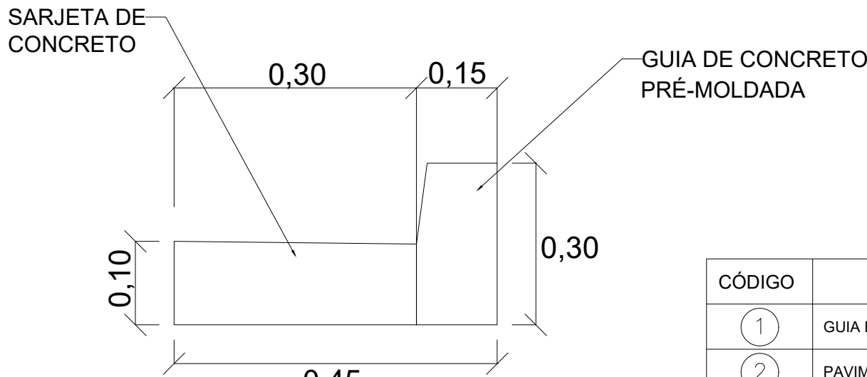
DETALHE A: GUIA E SARJETA DE CONCRETO SEM ESCALA
