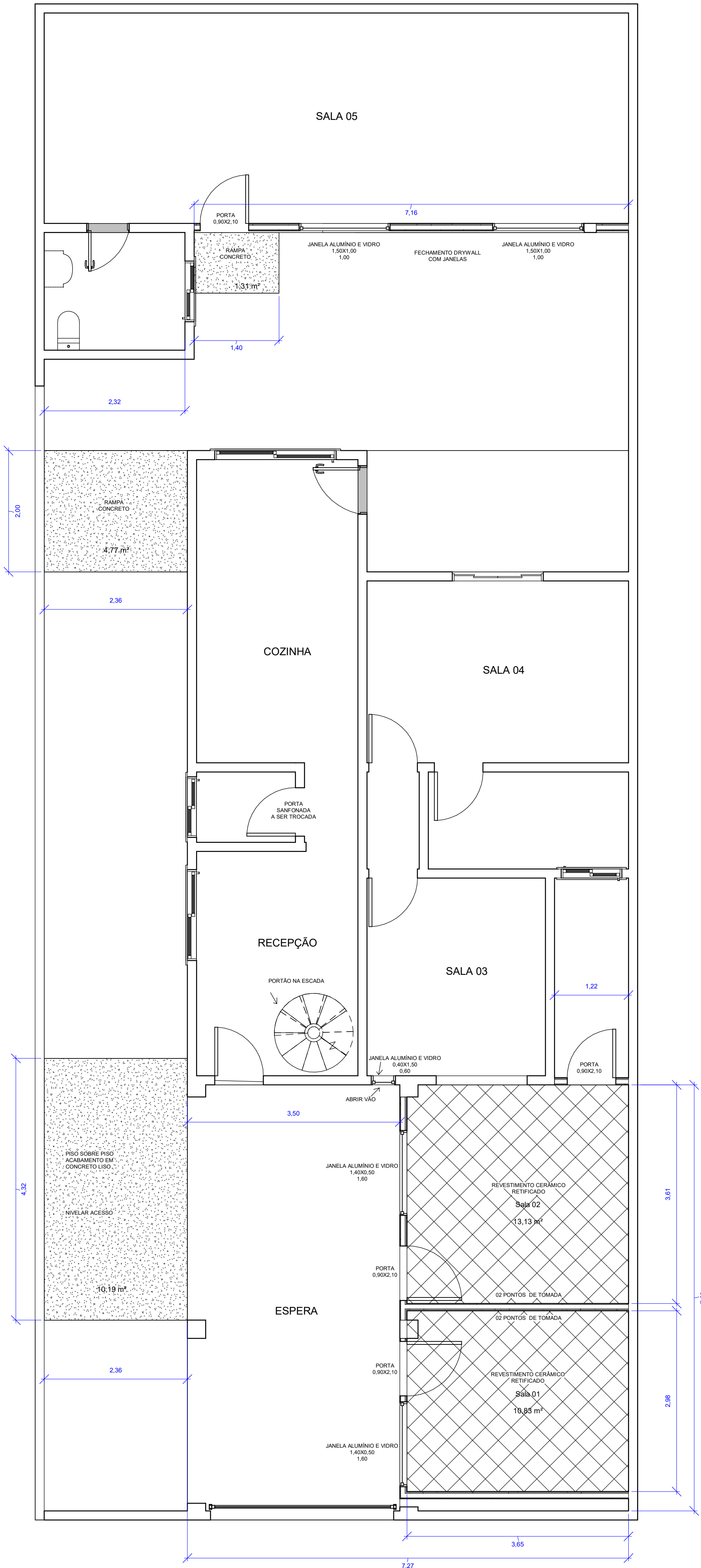
1 Piso inferior 1 : 50
