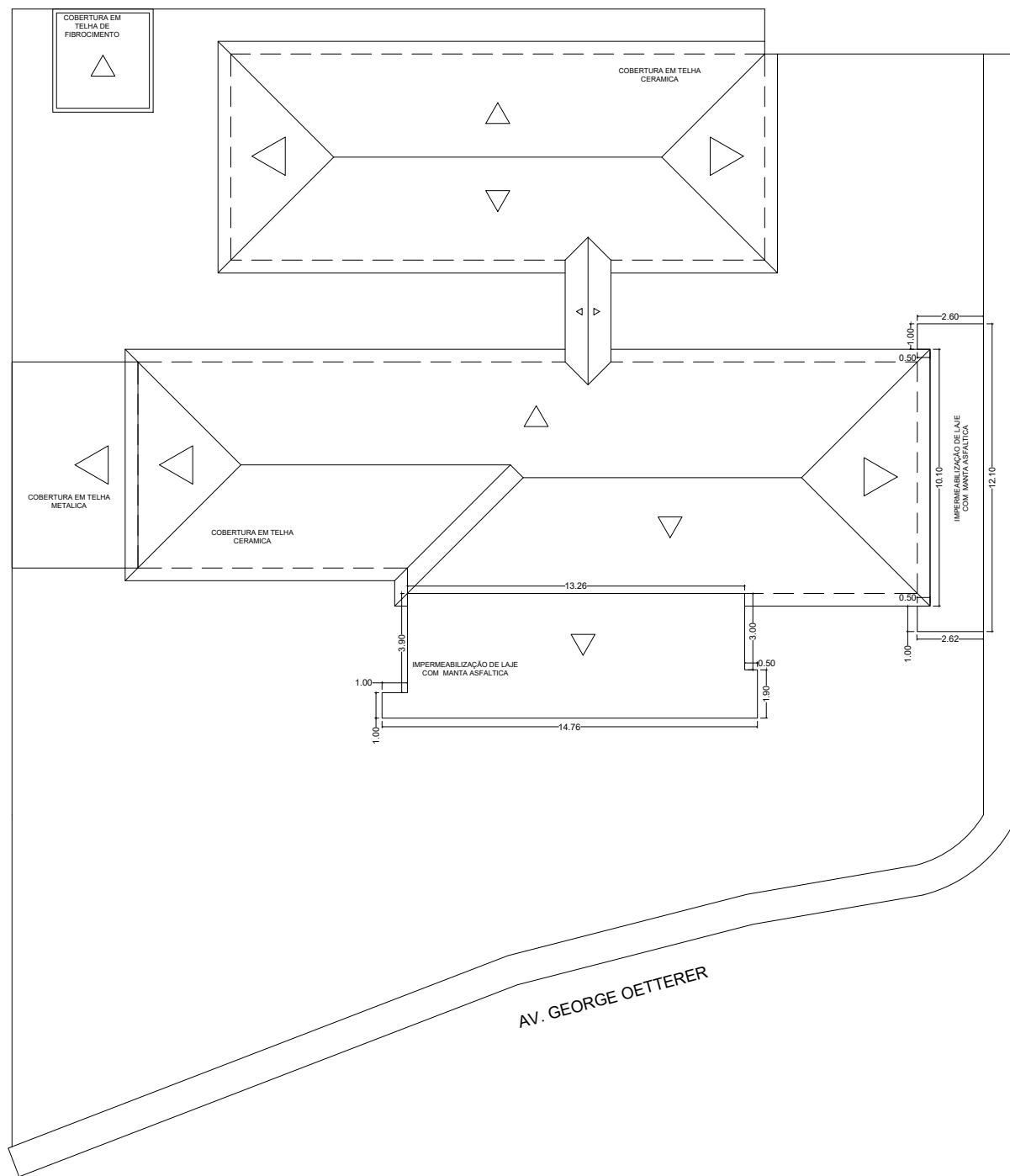
PLANTA DE COBERTURA ESC.: 1:250
