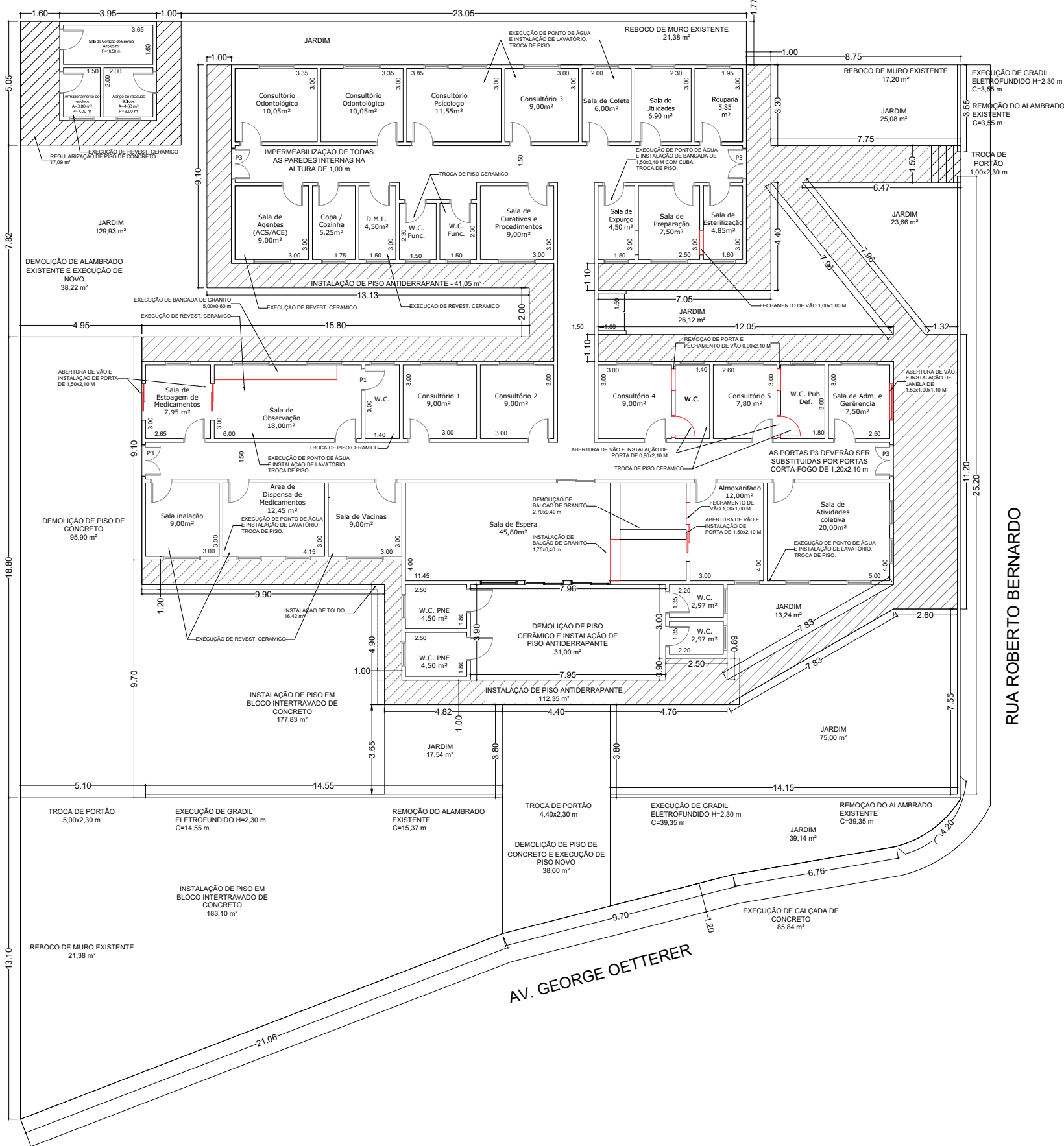
PLANTA BAIXA ESC.: 1:200
