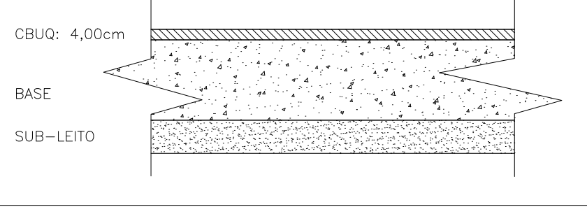
SECÇÃO TÍPICA DE PAVIMENTO ASFÁLTICO CBUQ
