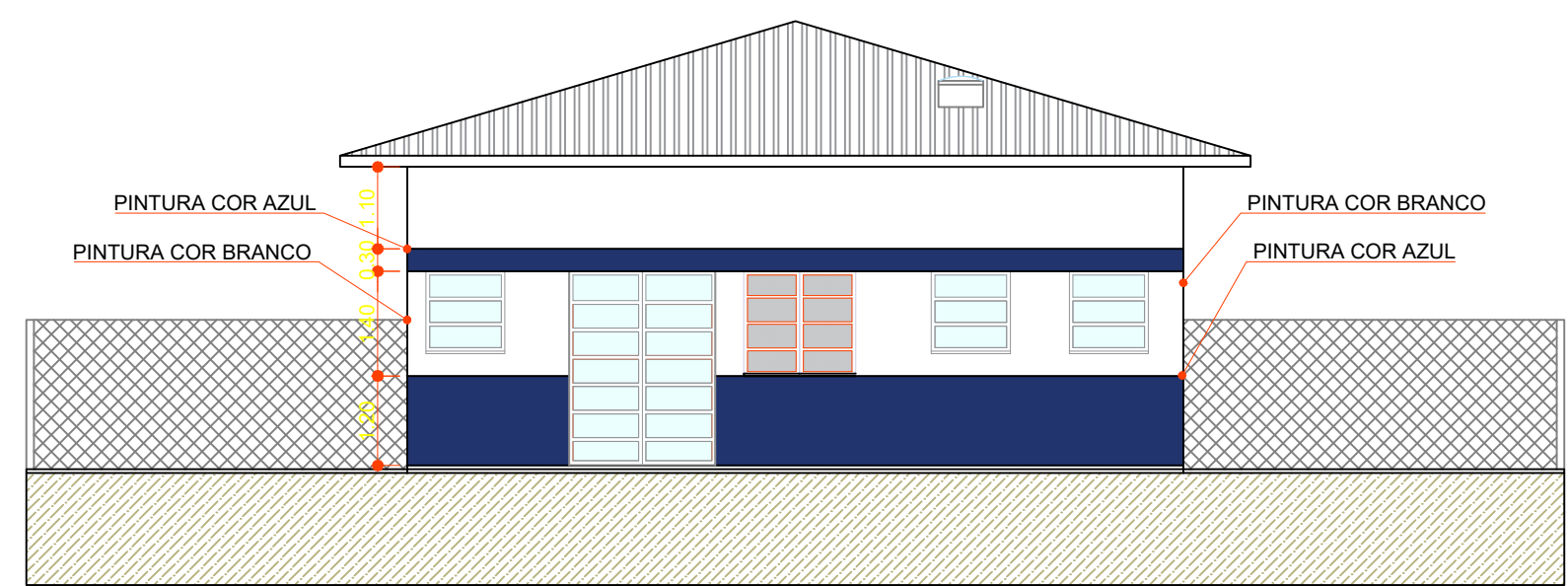
ELEVAÇÃO FRONTAL -01 ESCALA 1:100
