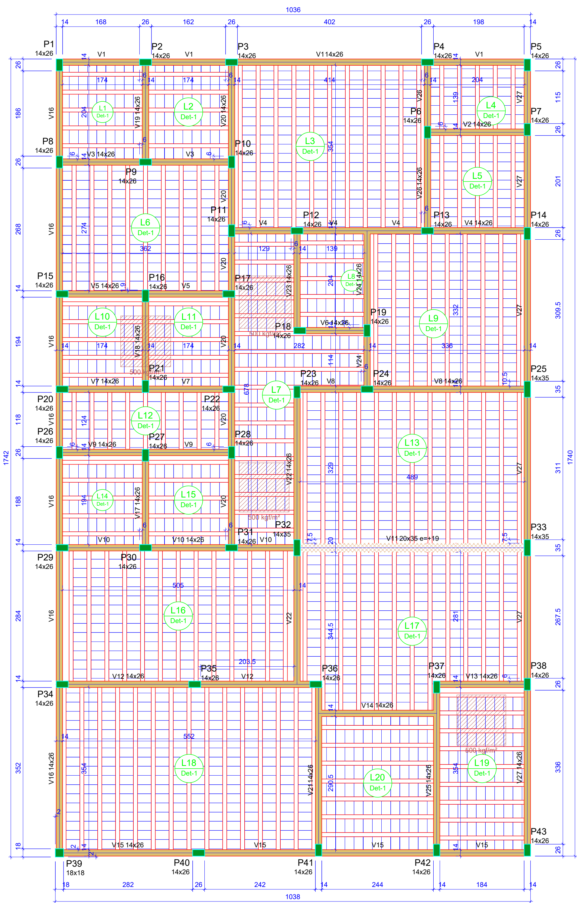
Locação do Terreo Escala 1:50
