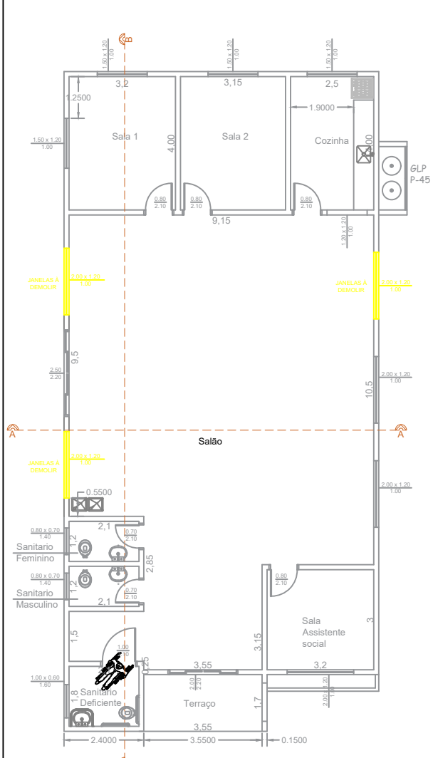
PLANTA DEMOLIÇÃO Escala 1:100
