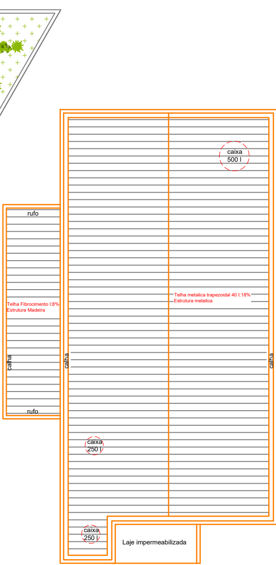
PLANTA DE COBERTURA escala 1:100
