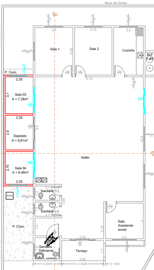
PLANTA AMPLIAÇÃO Escala 1:100
