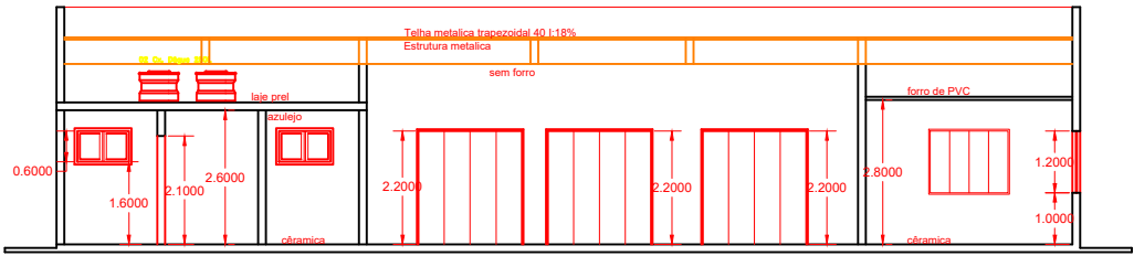
CORTE BB escala 1:100
