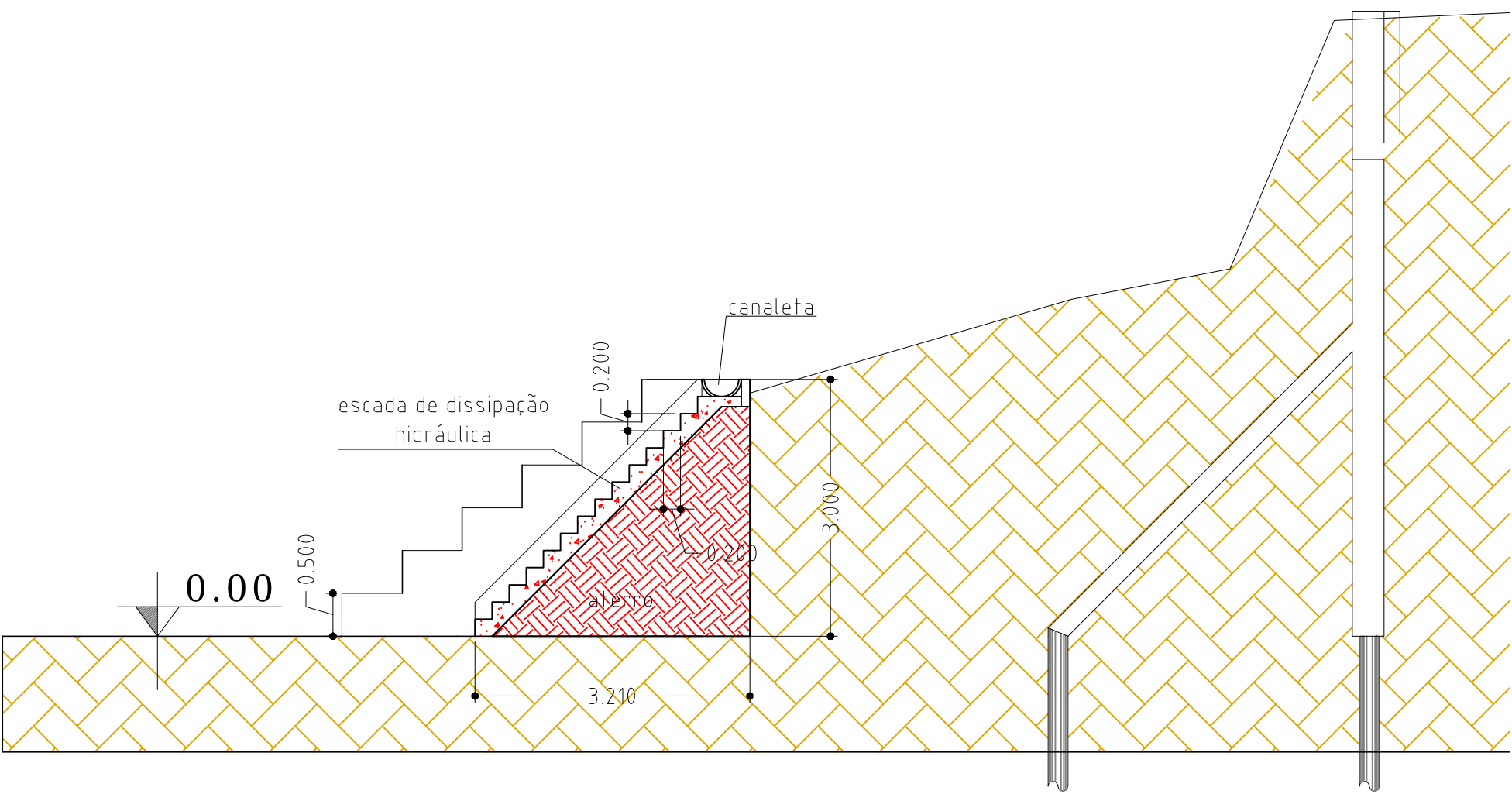
DET. ESCADA DE DISSIPÇÃO esc. 1:75
