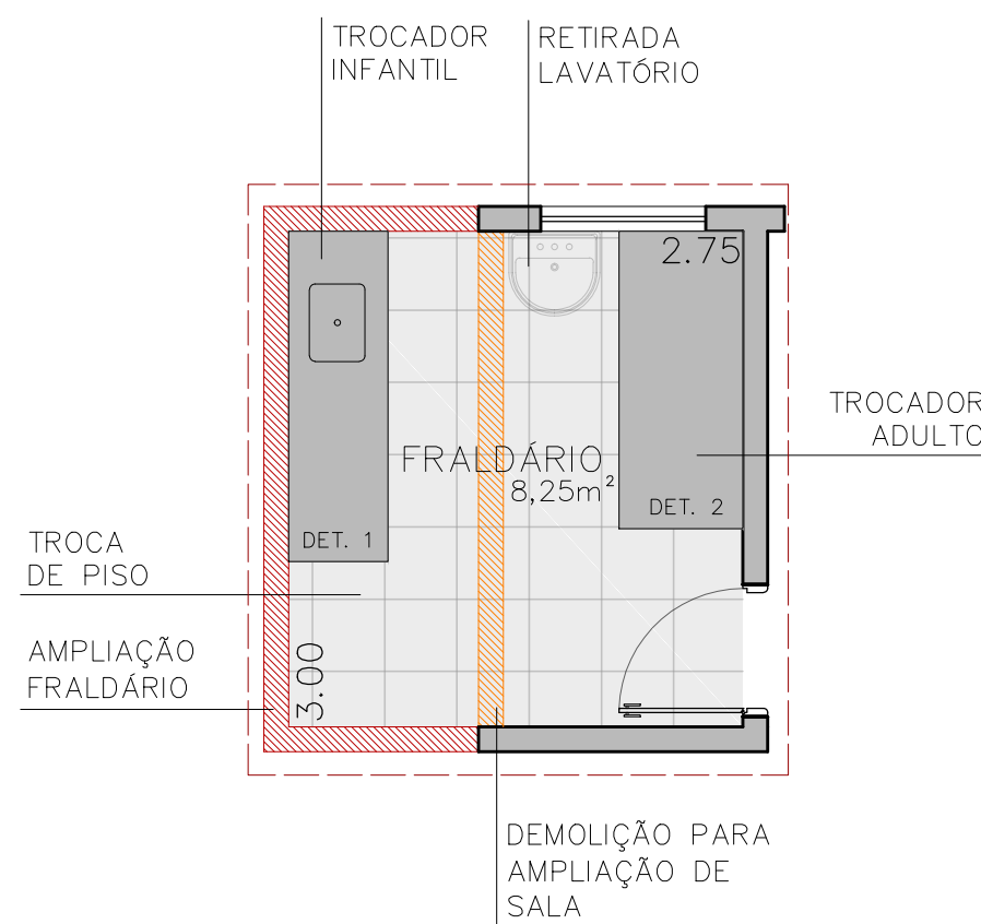
DETALHAMENTO FRALDÁRIO Esc.: 1/50
