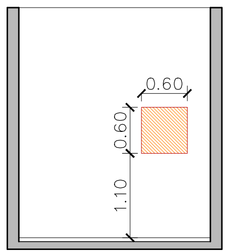
DETALHAMENTO VÃO DE PASSAGEM Esc.: 1/50
