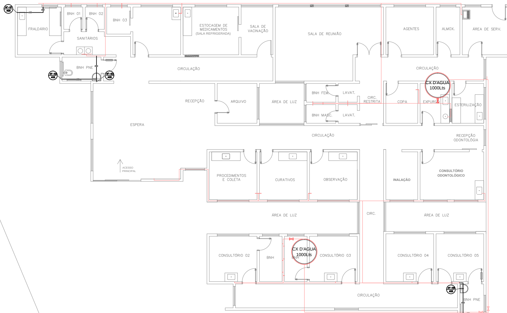
HIDROSSANITARIO - COBERTURA ESCALA 1:100
