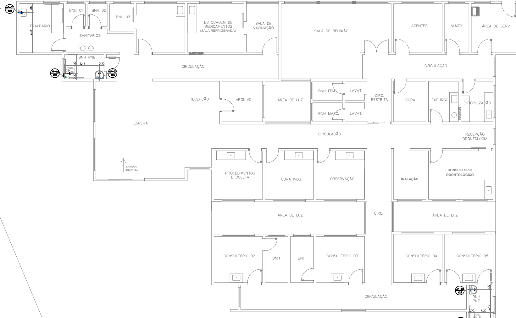
HIDROSSANITARIO ESCALA 1:100
