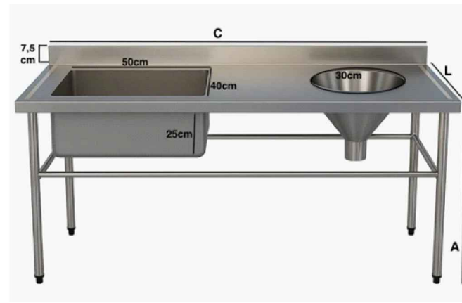
MOD. REFERÊNCIA BANCADA EXPURGO + CUBA 1,80m larg. x 0,60m prof. x 0,90 alt.
