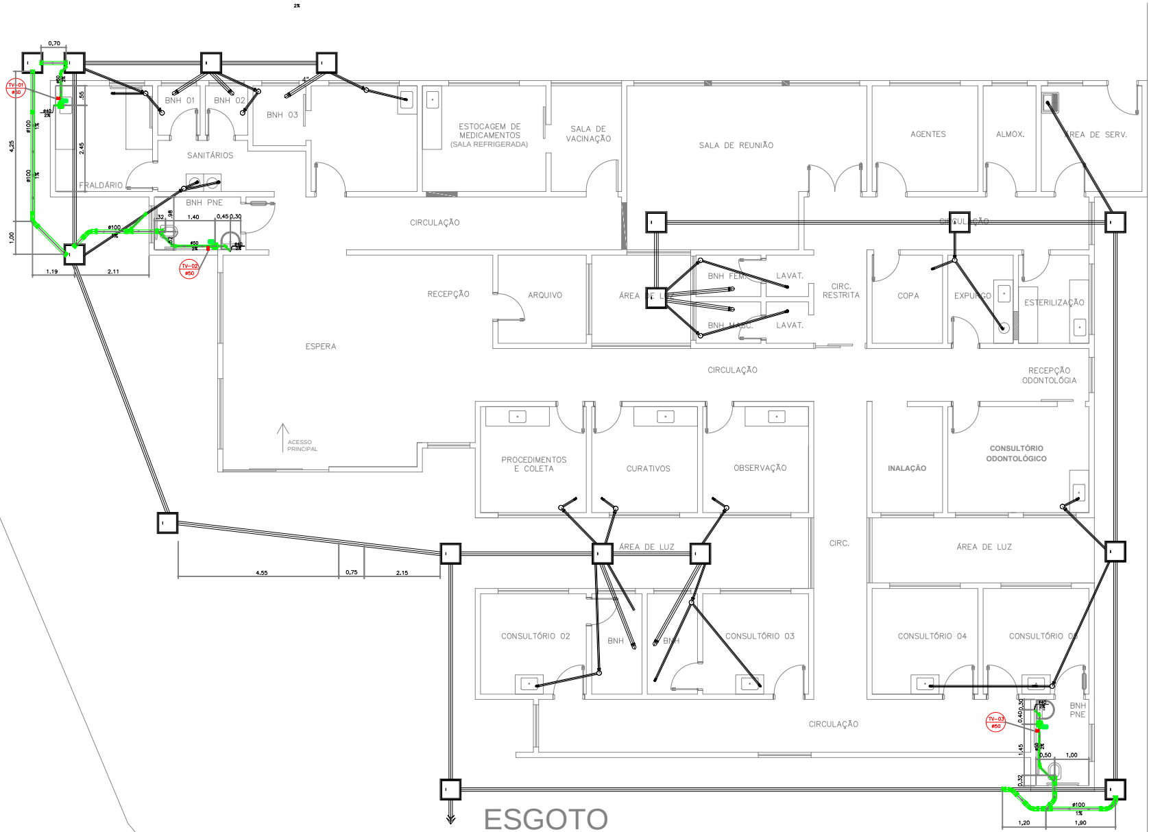
ESGOTO ESCALA 1:100
