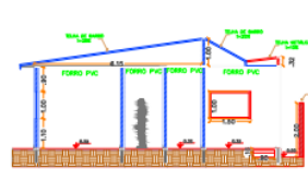
2 Corte B - B Escala 1/100
