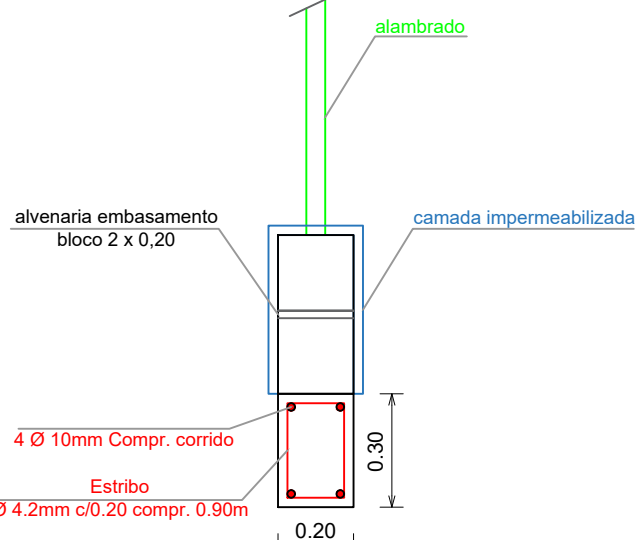
DET. VIGA BALDRAME ESC 1:20
