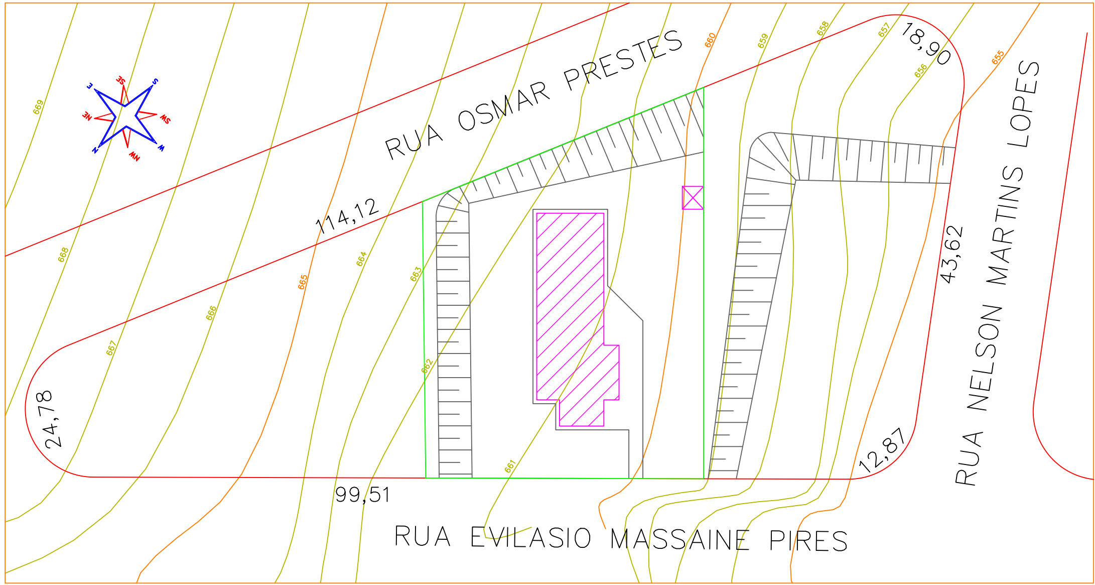
IMPLANTAÇÃO ESC: 1 / 500
