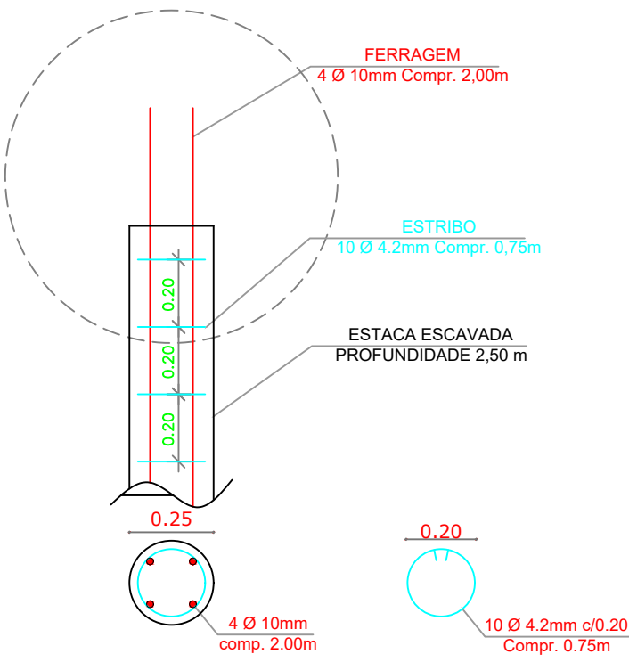
DET. BROCA CONCRETO Ø 25cm ESC 1:20
