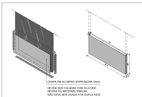
Figura 3 - detalhe chapa metálica para portas de madeira
