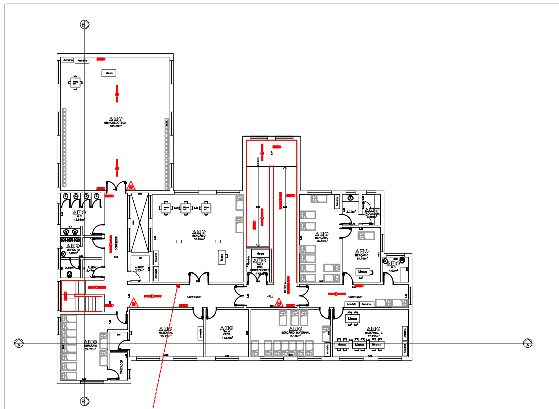
PLANTA BAIXA 1º PAVIMENTO ESC. 1:100
