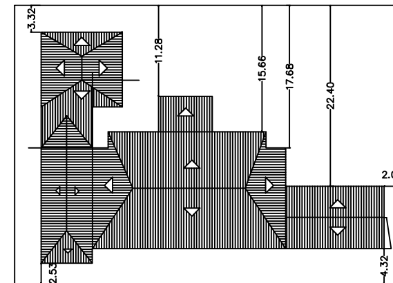
PLANTA DE COBERTURA SEM ESCALA
