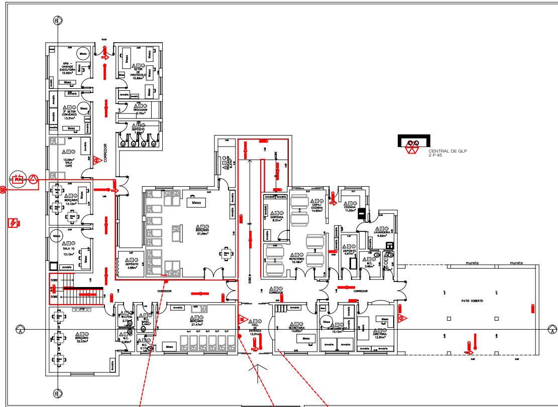
PLANTA BAIXA TÉRREO ESC. 1:100
