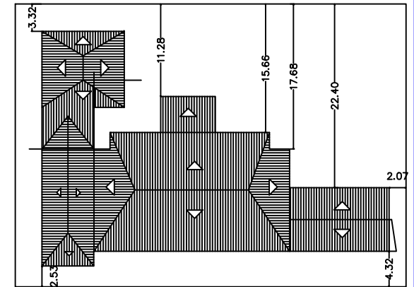
PLANTA DE COBERTURA SEM ESCALA
