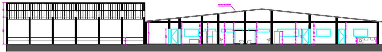
CORTE AA ESC.: 1:100
