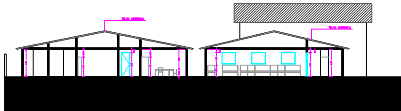
CORTE B ESC. 1:100
