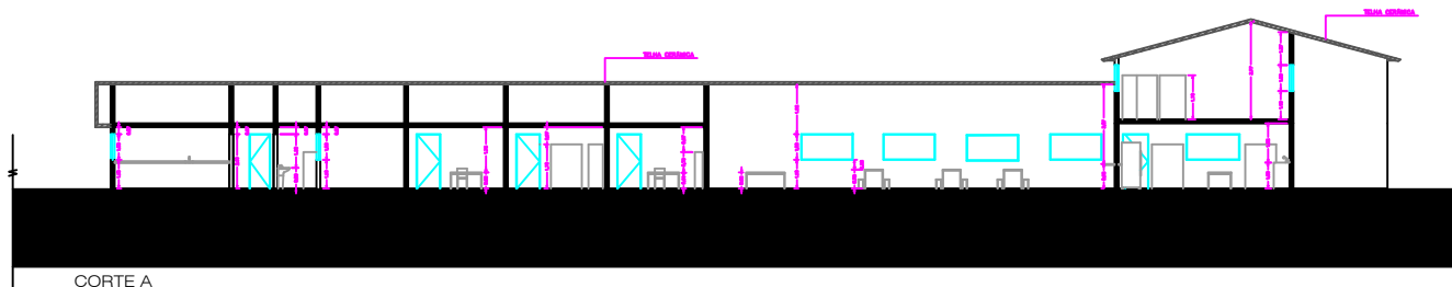
CORTE A ESC. 1:100
