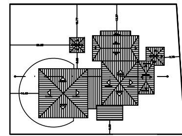
PLANTA DE COBERTURA SEM ESCALA
