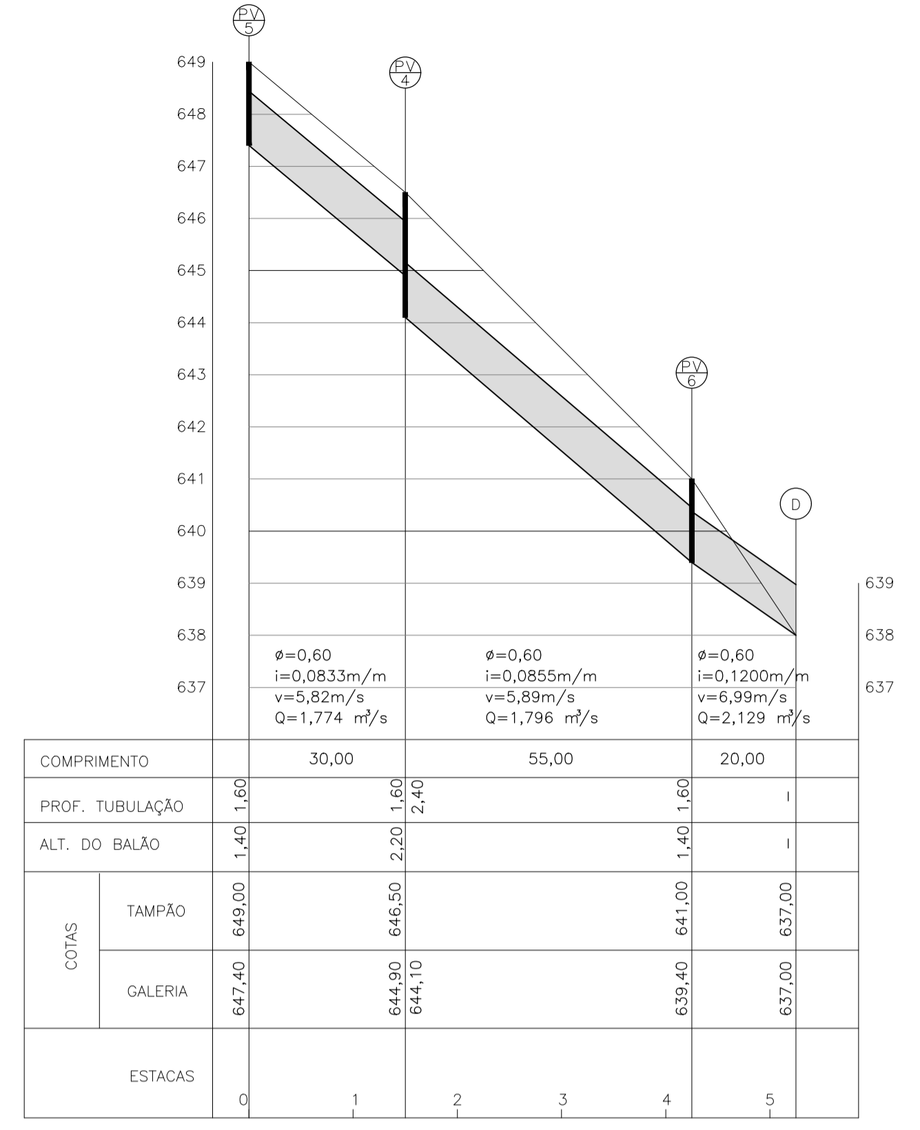
PERFIL LONGITUDINAL DA GALERIA - RUA DAS ROSAS ESC. H: 1:1.000 V: 1: 100
