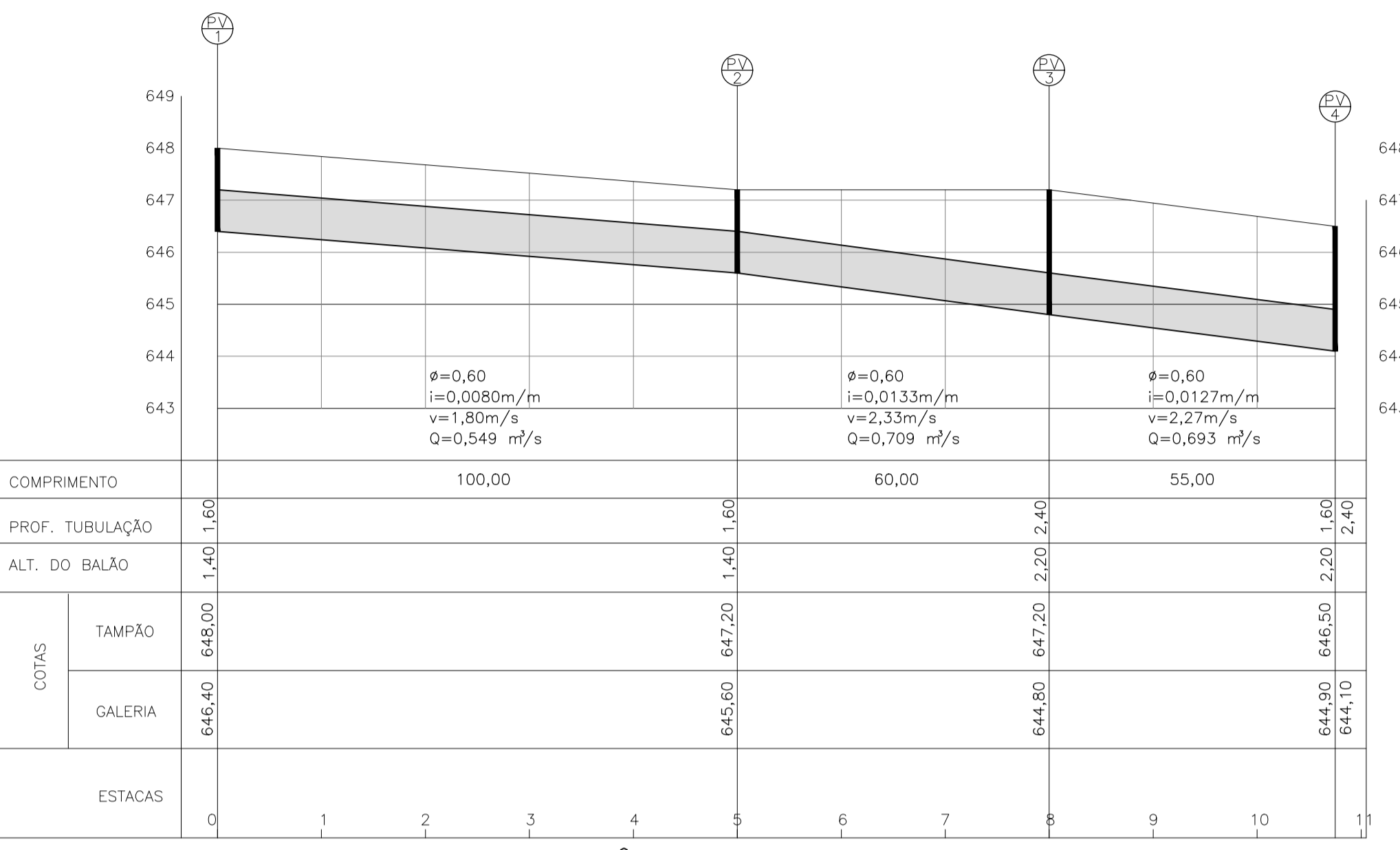
PERFIL LONGITUDINAL DA GALERIA - RUA DAS CALÊNDULAS ESC. H: 1:1.000 V: 1: 100
