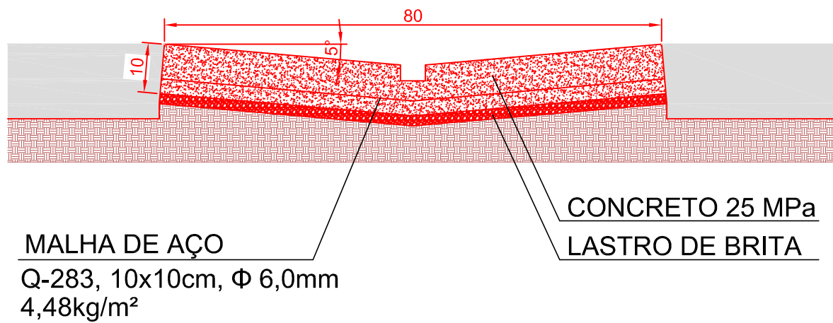
SEÇÃO TÍPICA DO SARJETÃO SEM ESCALA - MEDIDAS EM CM
