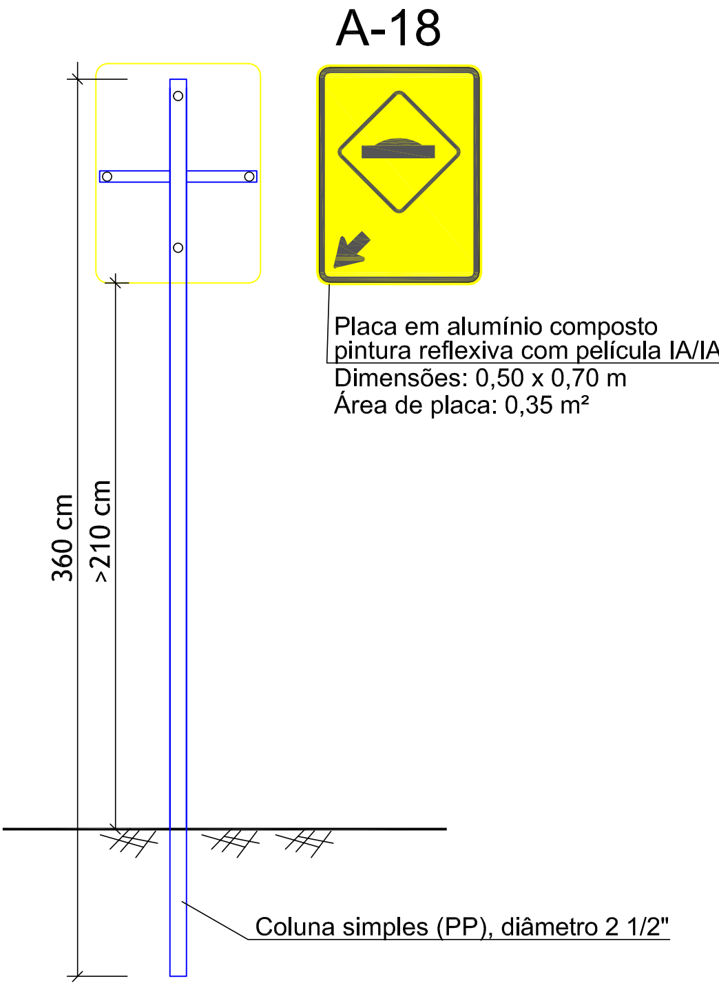
DETALHE SINALIZAÇÃO VERTICAL SEM ESCALA
