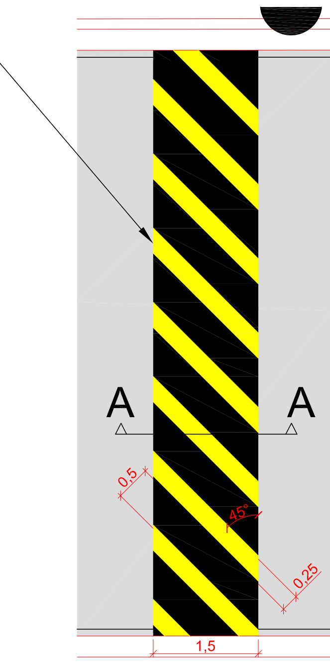
Seção transversal da lombada: 0,08m²
