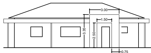
FACHADA ESC. 1:100
