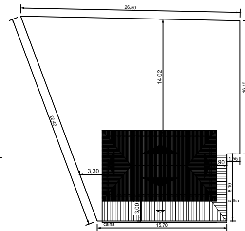
TERRENO E COBERTURA ESC. 1:200
