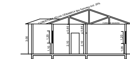
CORTE A.A ESC. 1:100
