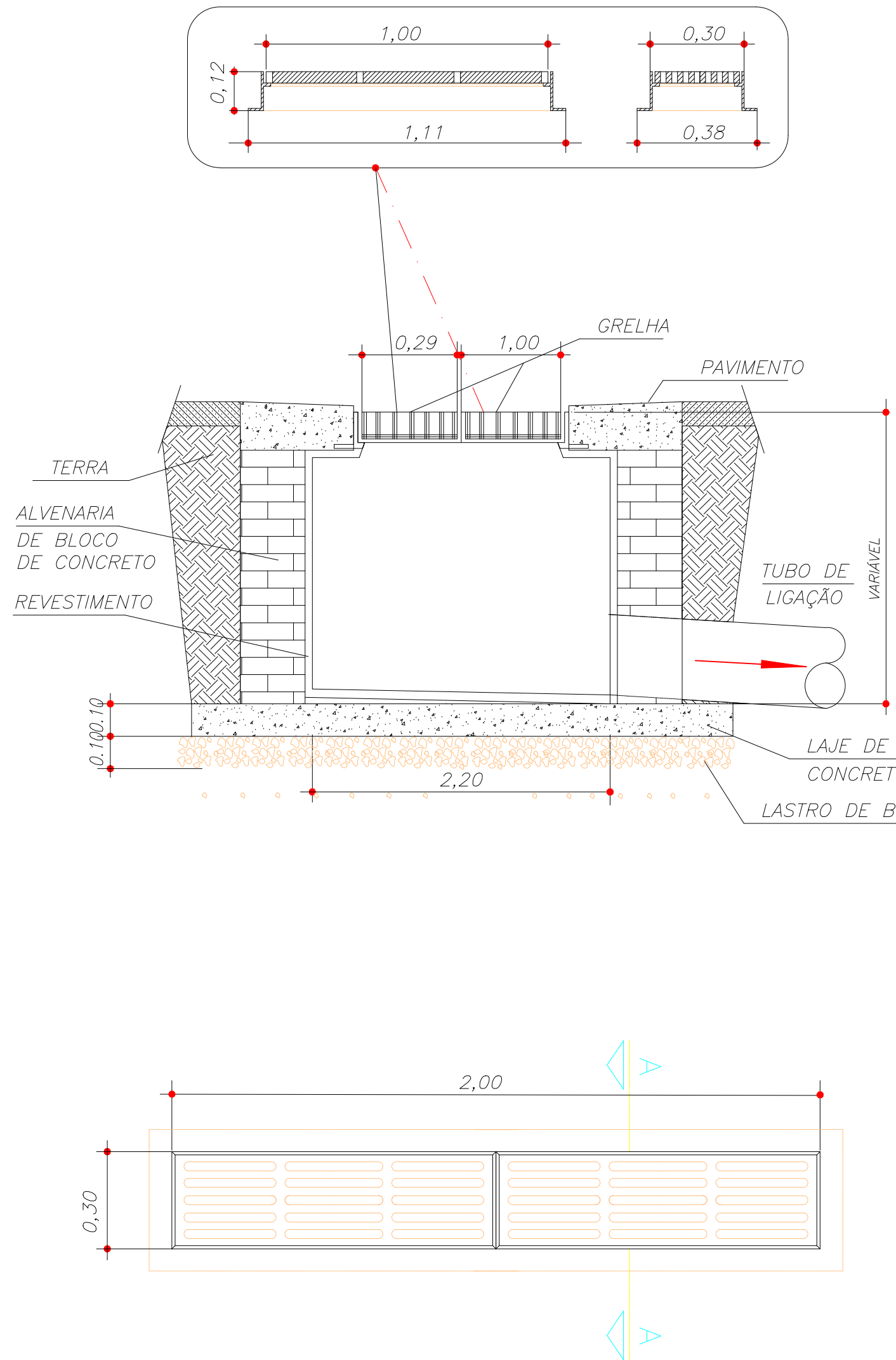
CORTE A-A
