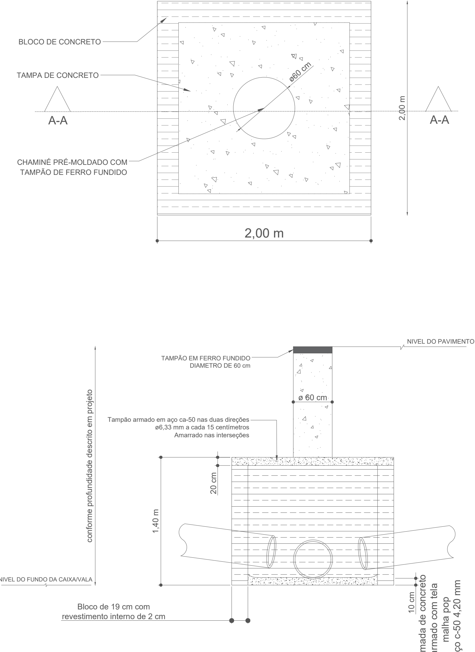
CORTE A-A
