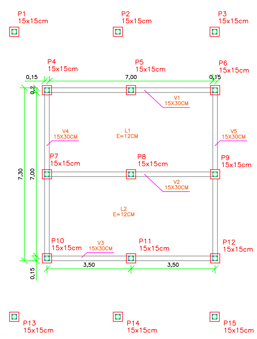
FORMAS 1:100
