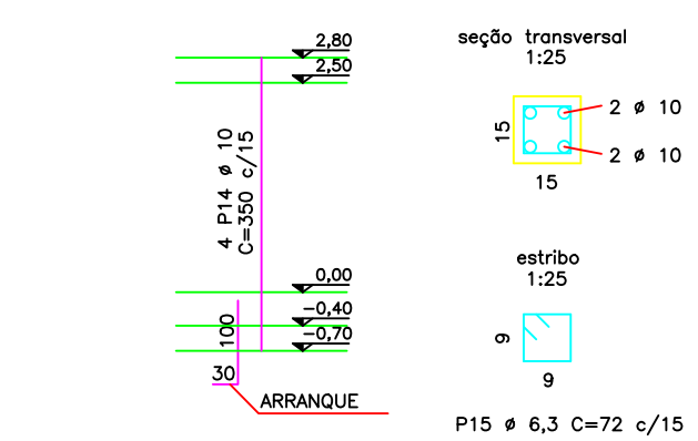
PILAR (15X) 1:100
