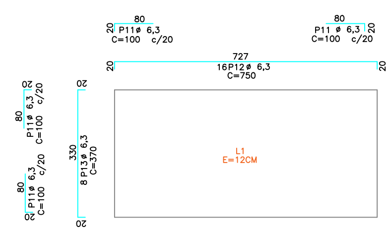
L1=L2 1:100
