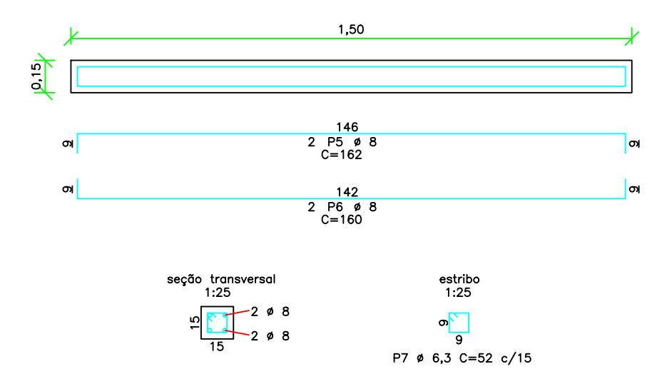
Verga/Contraverga (Janelas)
