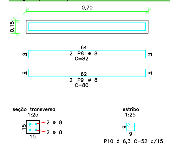
Verga (Portas)
