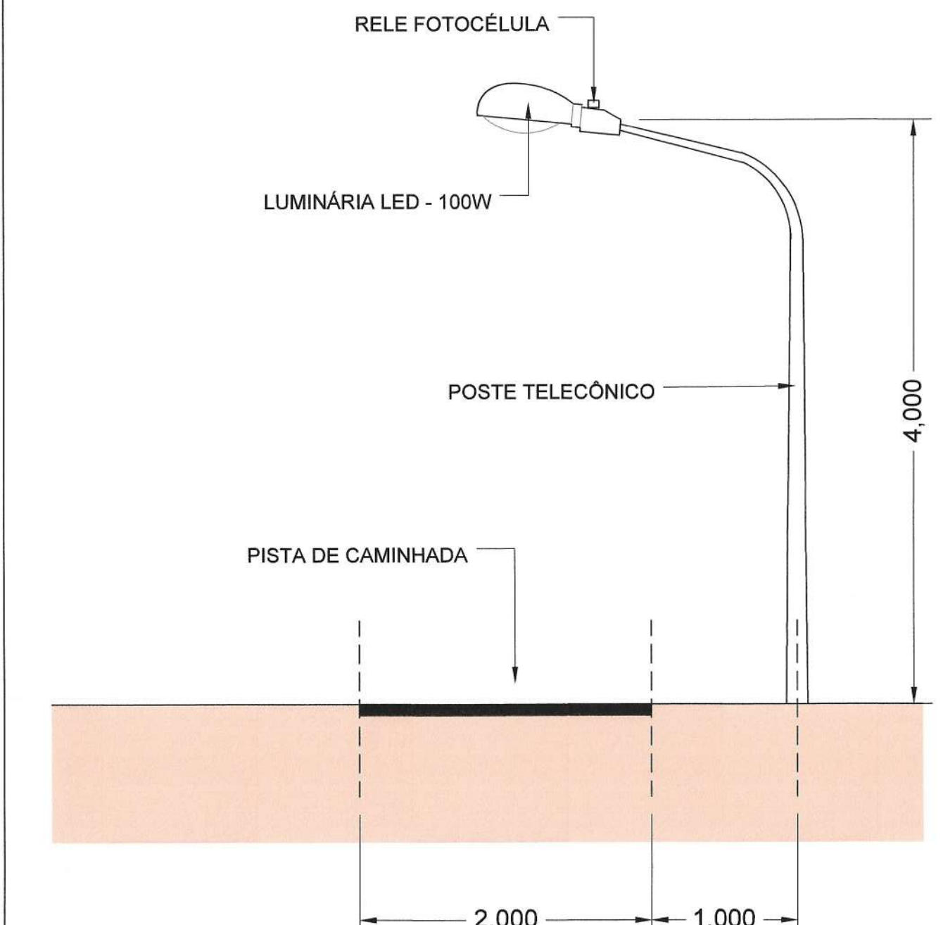
DETALHE DO POSTE SEM ESCALA - MEDIDAS EM M
